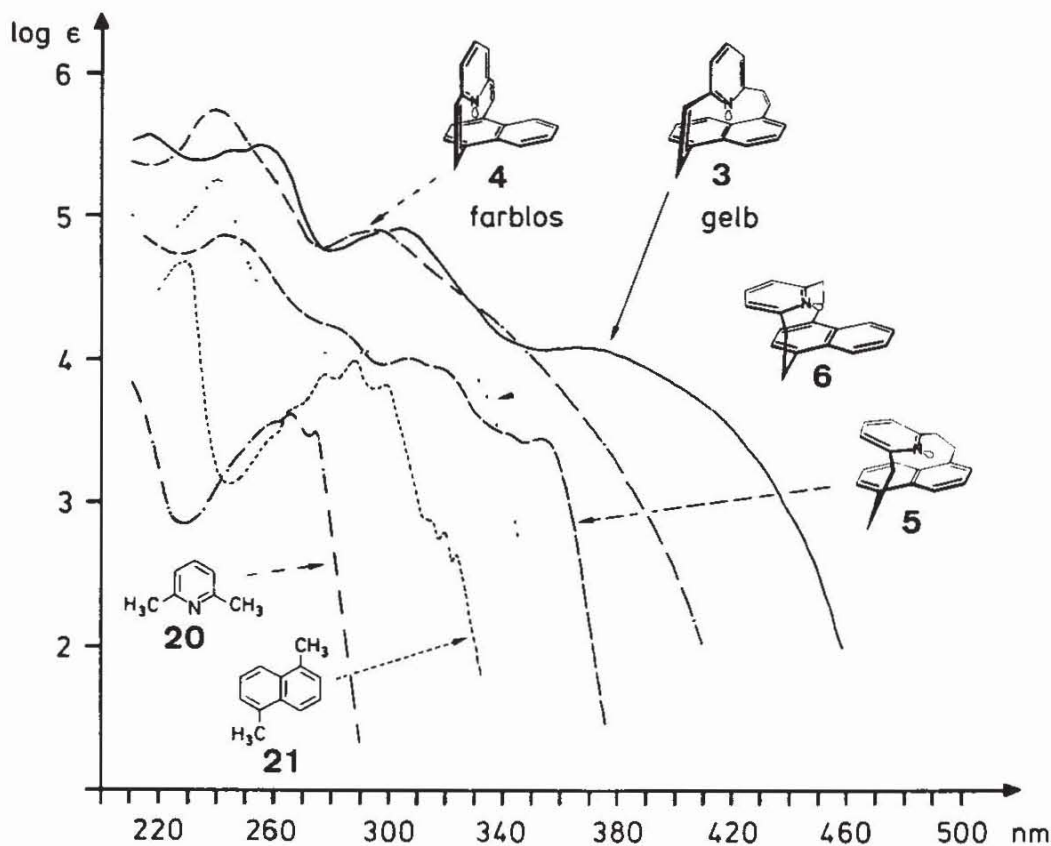
Abb. 7. UV-Absorption (in Cyclohexan, Raumtemp.) von 3–6 im Vergleich zu 2,6-Dimethylpyridin (20) und 1,5-Dimethylnaphthalin (21). Die Spektren von 5, 6 und 3, 4 sind um 0,5 bzw. 1 Ordinateneinheit verschoben
