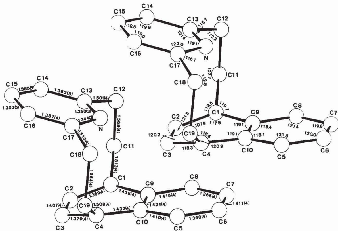
Abb. 6. Molekülstruktur, Bindungslängen (Å) und -winkel (°) von 6
