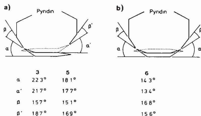
Abb. 5. a) Deformation der Naphthalin-Einheiten in 3 und 5
