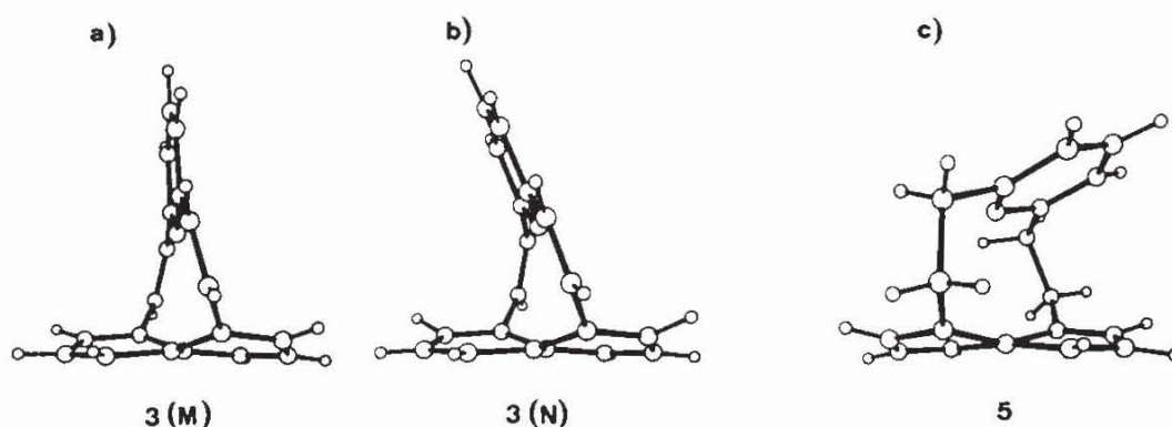
Abb. 2. Orientierung des Pyridin-Ringes relativ zur Naphthalin-Einheit in 3 und 5 . a) und b): Die beiden unabhängigen Moleküle M und N von 3 . c): Erstes unabhängiges Molekül von 5 ; das zweite unterscheidet sich nicht merklich und ist nicht abgebildet
