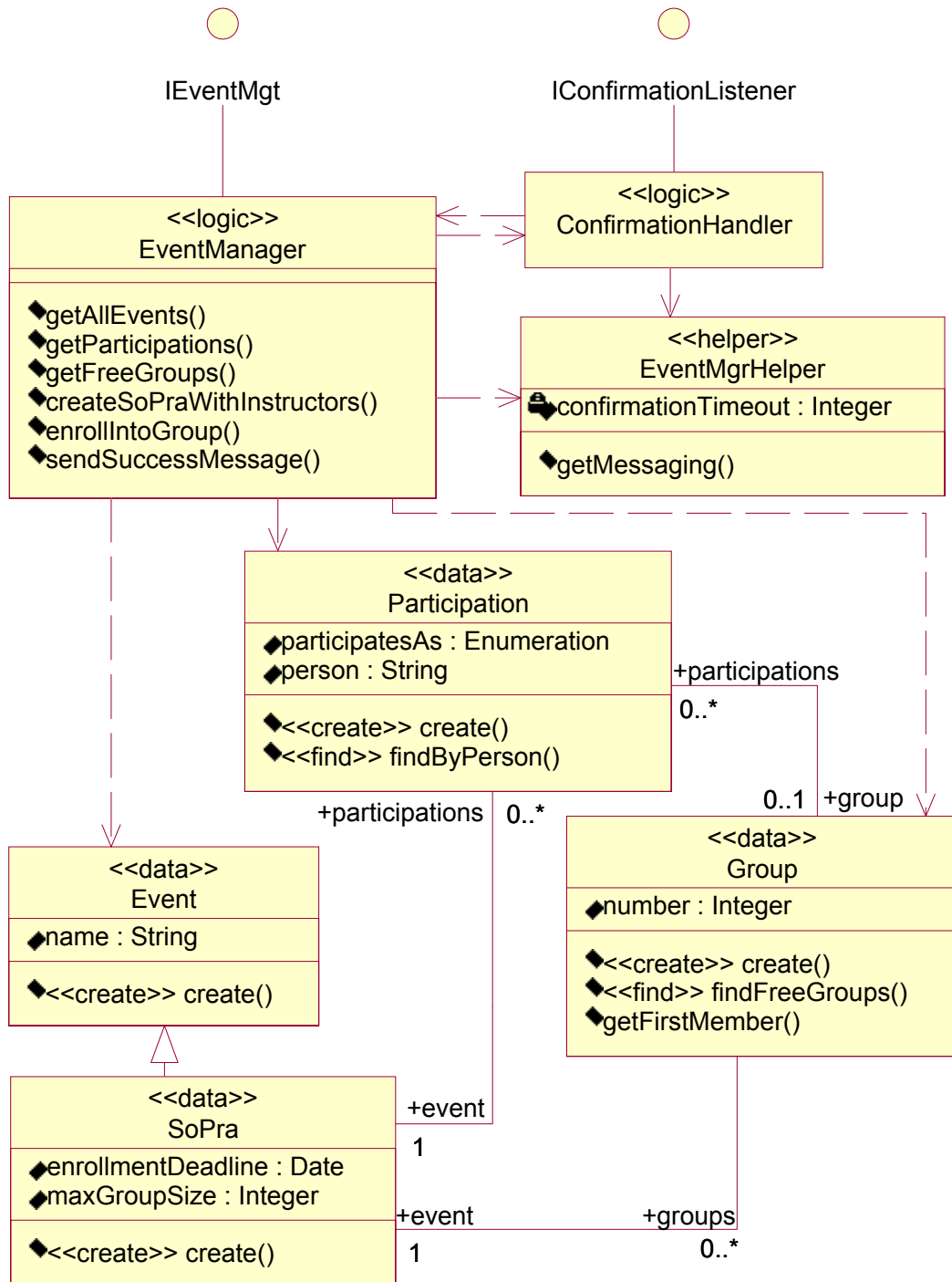
Abbildung 6.8: Entwurf der Komponente EventManagement
