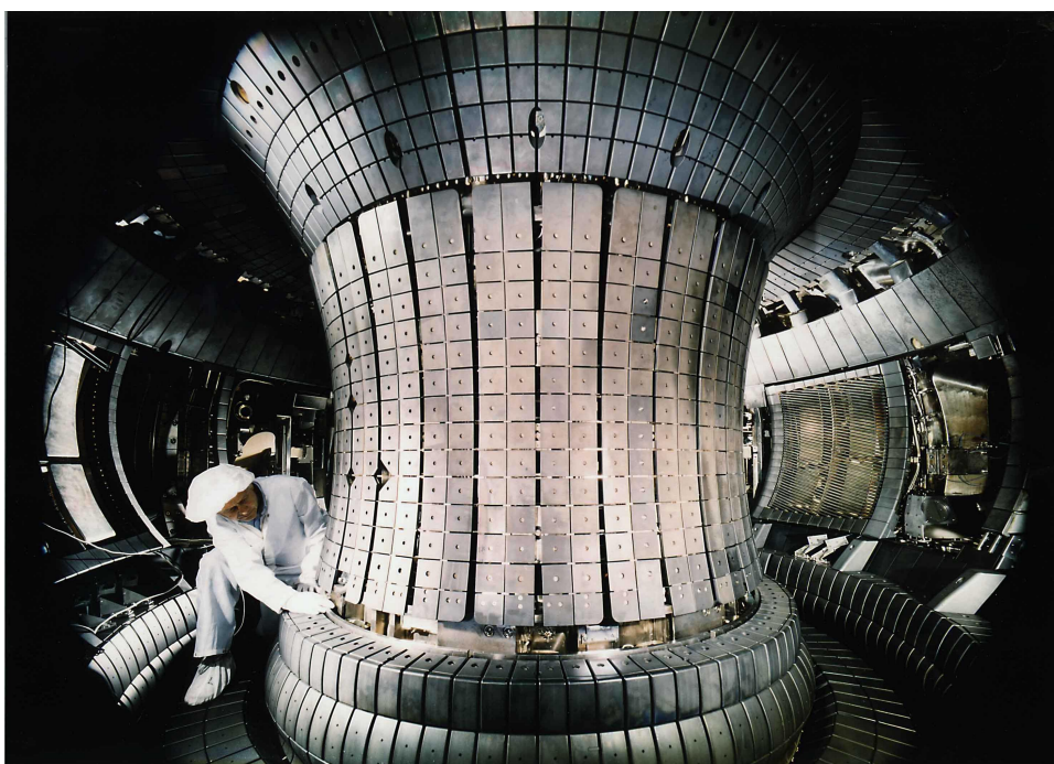
Abbildung 3: Blick in das Vakuumgefäß des Experimentalreaktors „Asdex Upgrade“ im Max-Planck-Institut für Plasmaphysik in Garching bei München
