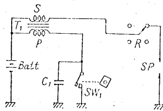
Abb.1 Das bisher gebräuchliche Kontaktsystem
