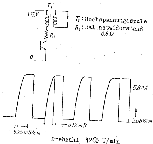
Abb.13 Die Primärstromwellenform
