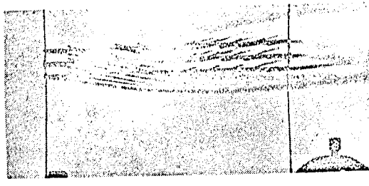
(A) Schlieren-Aufnahme erhitzter Modellrippen, im Windkanal
