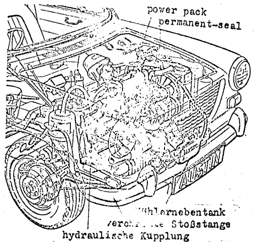
Abb.7 Das "Permanent-Seal" Verfahren des Austin 1100
