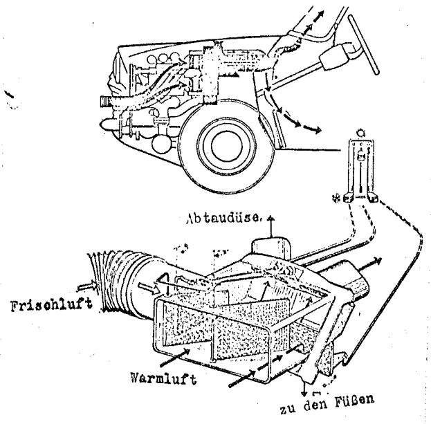
Abb.11 Der gleichzeitig als „Wagenheizer“ benützte Kühler des DKW F 12
