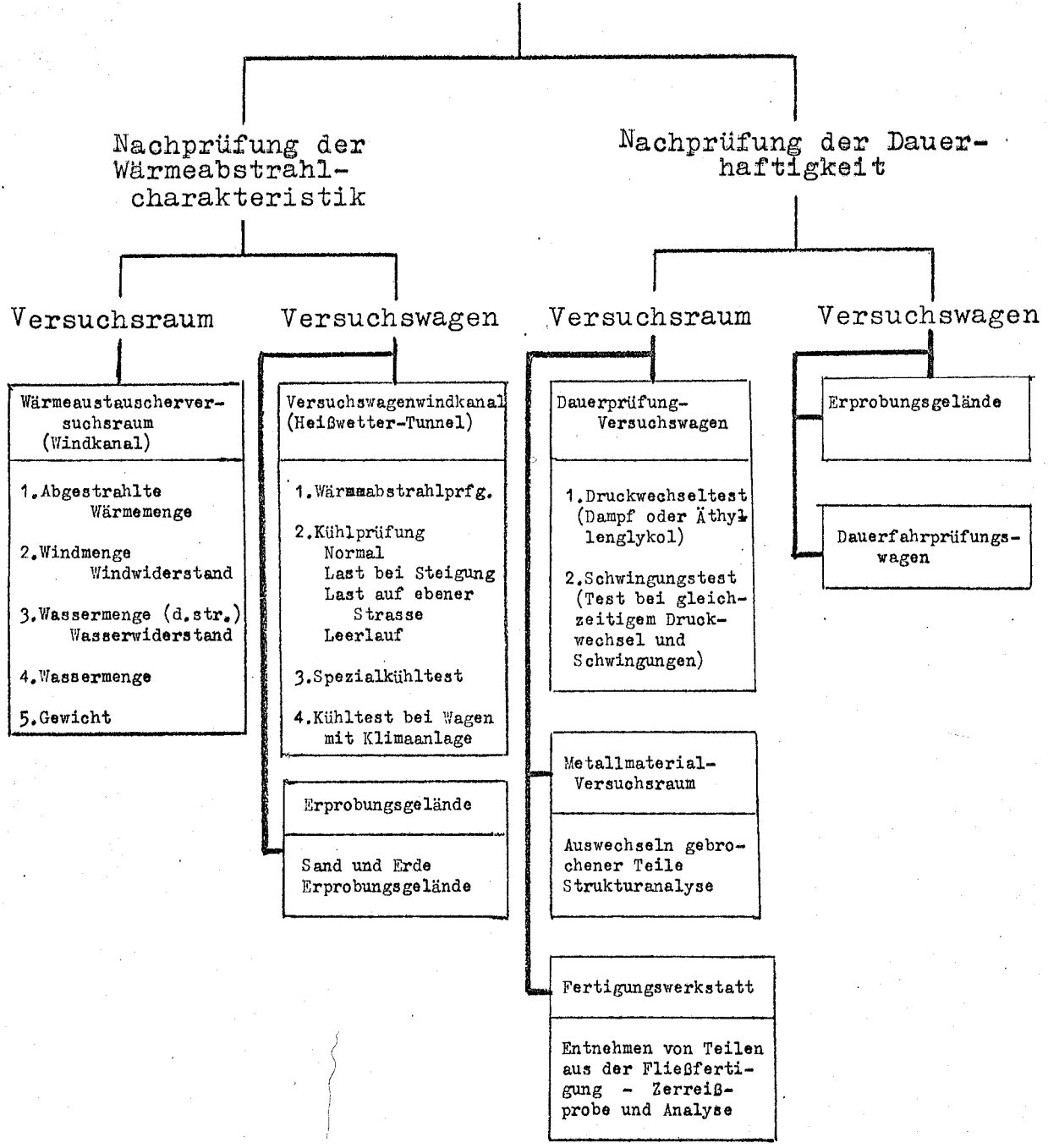
Abbildung 14. Kühlerprüfverfahren
