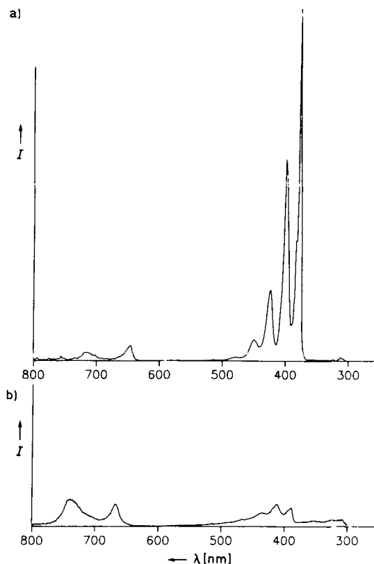
Abb. 2. Emissionsspektren ( n -Hexan, T=180 K, Anregung bei 257 nm) von a) Anthracen/5,10,15,20-Tetraphenylporphyrin (1/1), Konzentration 10^{-6} mol L ^{-1} (das Spektrum entspricht einer Überlagerung der Einzelspektren) und b) 3-A,TPP, Konzentration 2 \cdot 10^{-5} mol L ^{-1} (der Ursprung der schwachen Emission zwischen 300 und 380 nm ist noch nicht bekannt).
