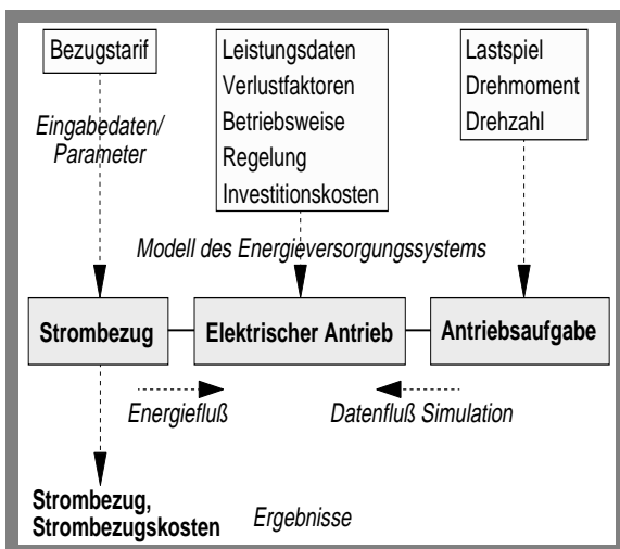
Abbildung 5: Datenfluß bei der Simulation von elektrischen Antrieben
