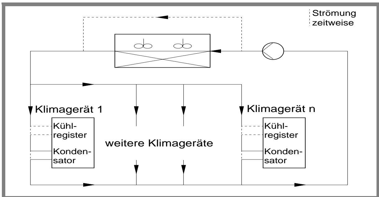
Abbildung 6: Schema des Rückkühlkreislaufts
