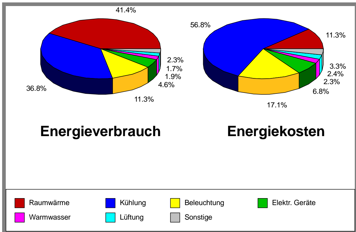
Abbildung 2: Typischer Zusammenhang zwischen Energieverbrauch und -kosten im Lebensmitteleinzelhandel: Ergebnis von Betriebsbegehungen
