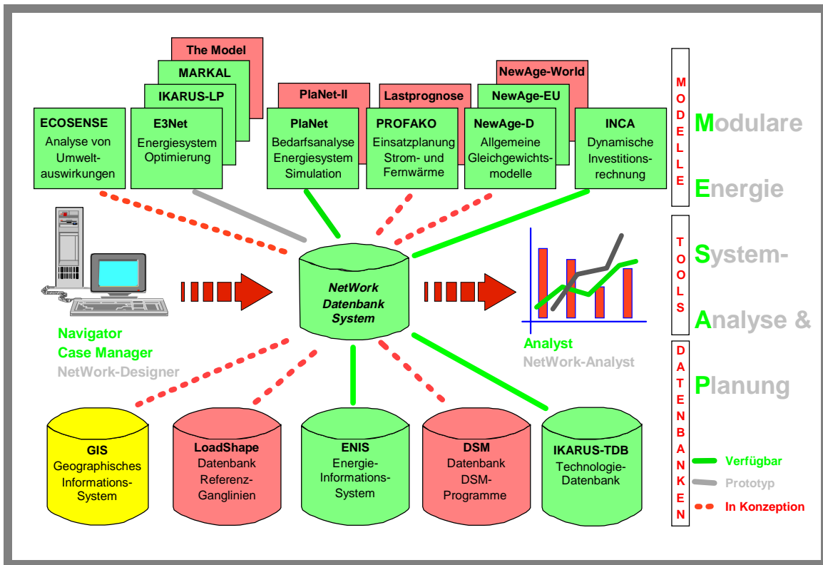
Abbildung 1: Modulares Energieplanungs- und Analysesystem MESAP
