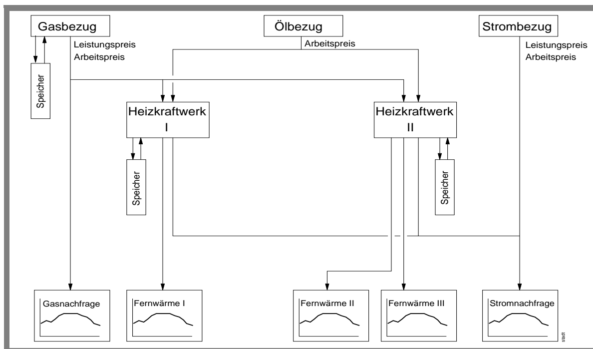
Abbildung 6: Vereinfachtes Modell des Kraftwerkssystems der Stadtwerke
