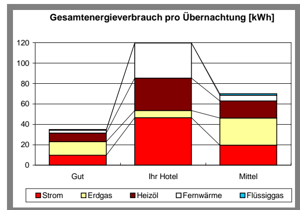
Abbildung 3: Energiebenchmarking: Einordnung eines individuellen Hotels im Verhältnis zu Branchenkennziffern
