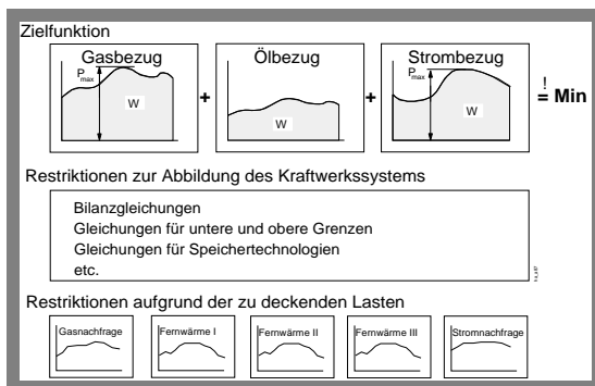
Abbildung 7: Optimierungsproblem der Einsatzplanung für das Kraftwerkssystem
