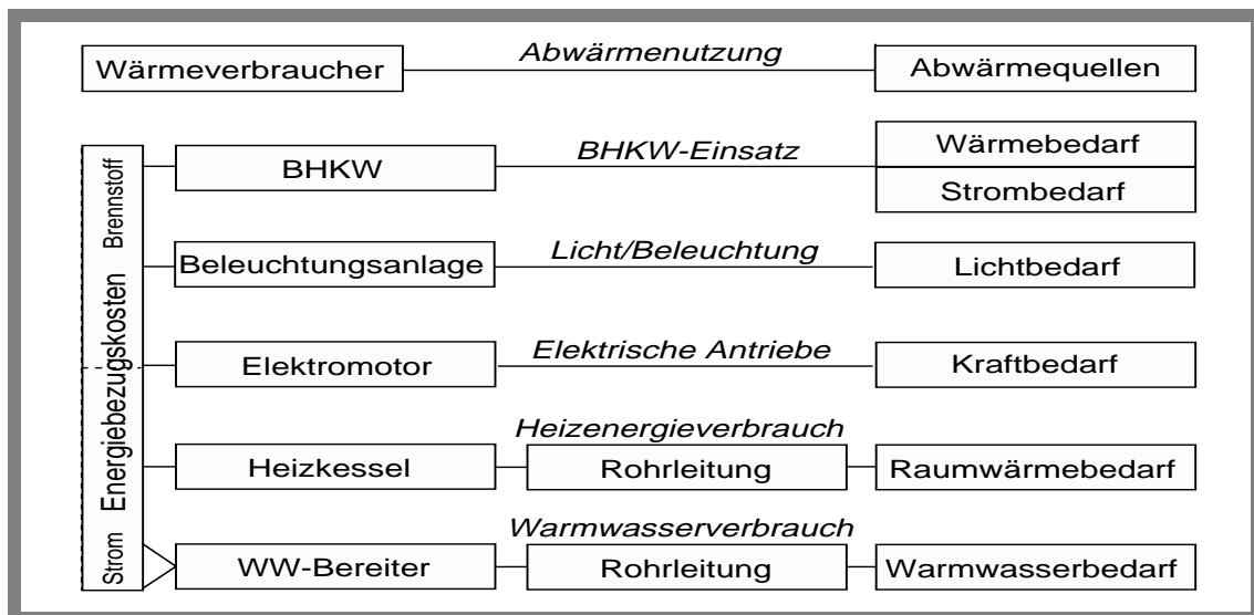
Abbildung 4: Anwendungsbereiche und Modellstruktur von MOSAIK
