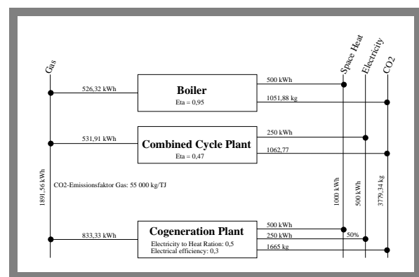
Abbildung 3: Beispiel für ein Referenzenergiesystem
