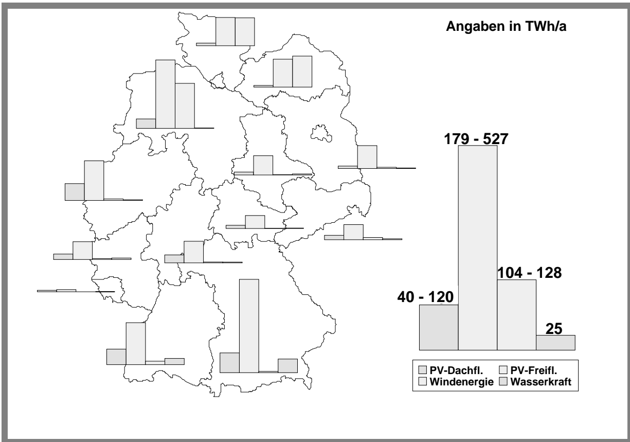
Abbildung 1: Technische Potentiale einer Stromerzeugung aus Wasserkraft, Windenergie und Solarstrahlung in der Bundesrepublik Deutschland
