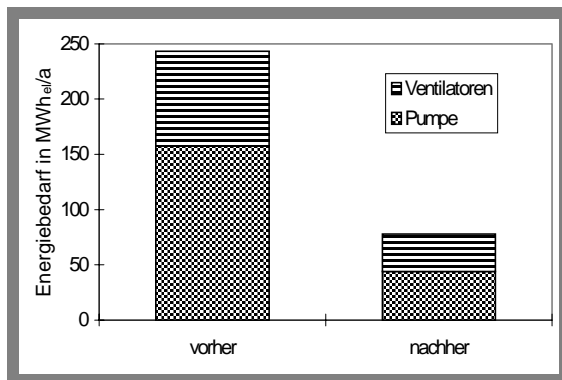
Abbildung 7: Energiebedarf Pumpen/Ventilatoren
