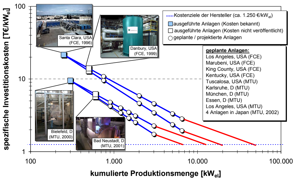
Abb. 2-22: Abschätzung der Erfahrungskurven für die MCFC-Systeme von FCE und MTU
