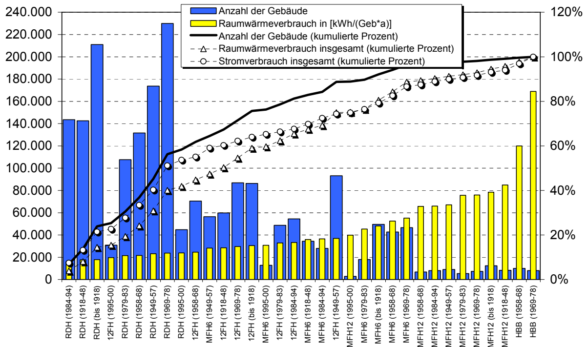
Abb. 3-13: Raumwärme- und Stromverbrauchsmatrix der Haushalte in Baden-Württemberg nach Gebäudetypen und -baualtersklassen
