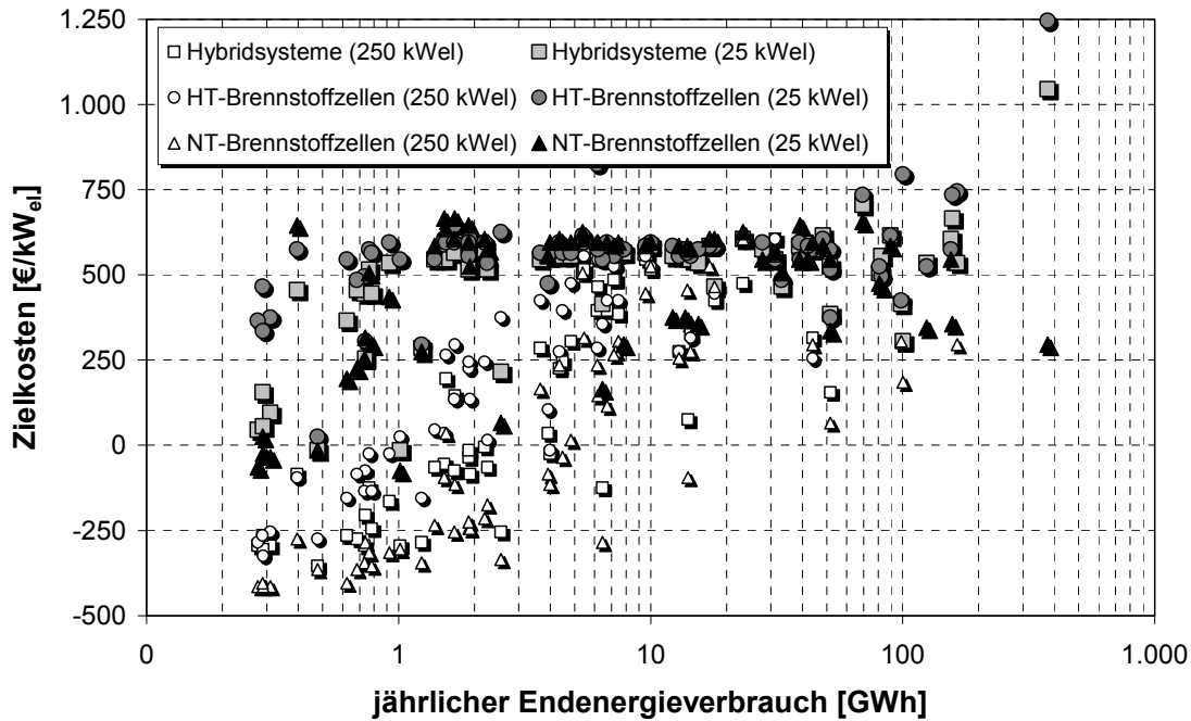
Abb. 4-17: Auswirkung einer angepassten Anlagenleistung in der Industrie am Beispiel einer Modulgröße von 25 kW eI im pessimistischen Preisszenario
