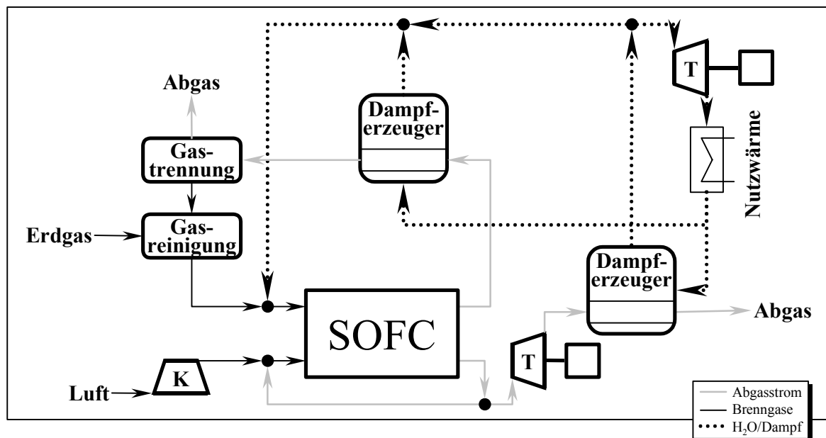
Abb. B-10: Flussschema eines SOFC-Hybridsystems (nachgeschalteter GuD-Prozess)
