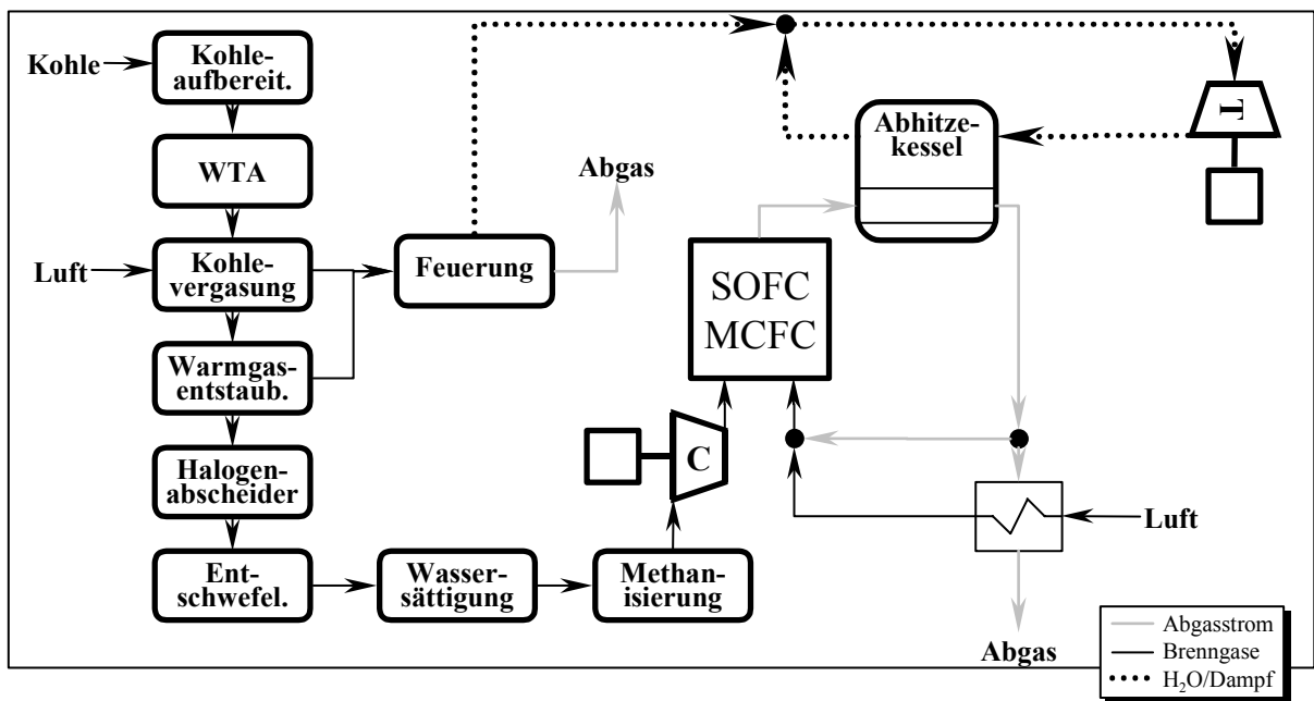
Abb. B-6: Flusschema der Kohleverstromung in Hochtemperatur-Brennstoffzellen
