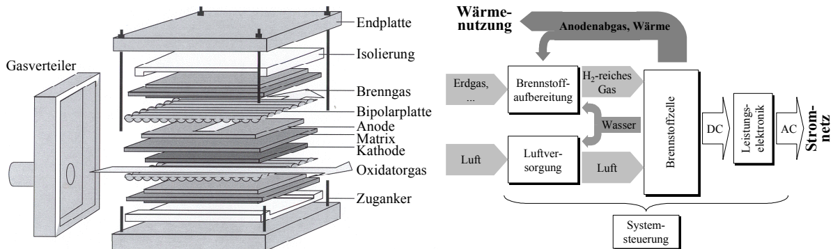
Abb. 2-3: Aufbau eines Brennstoffzellenstacks und schematische Darstellung des Systemaufbaus stationärer Brennstoffzellenanlagen
