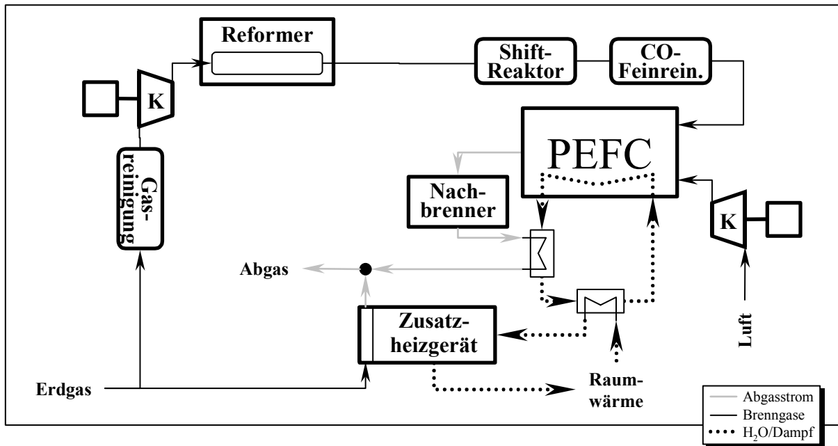
Abb. B-1: Flusschema eines Hausenergieversorgungssystems auf Basis der PEFC
