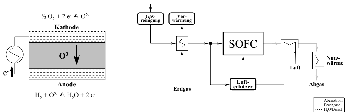
Abb. 2-9: Zellreaktionen der SOFC und Flussschema eines dezentralen SOFC-KWK-Systems
