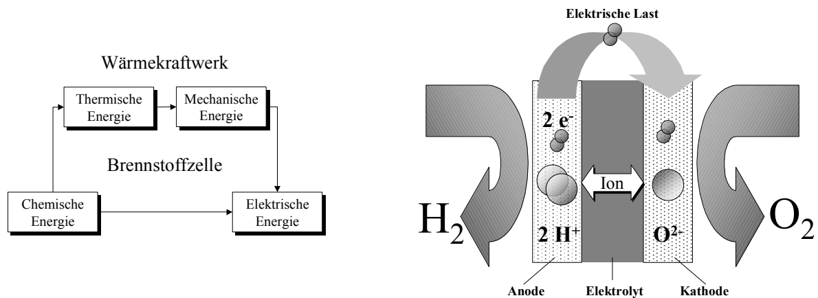
Abb. 2-1: Schematische Darstellung der direkten Energiewandlung in Brennstoffzellen
