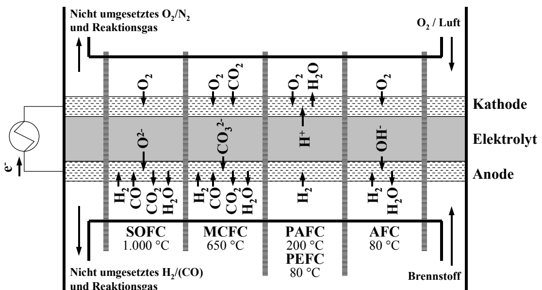
Abb. 2-4: Ionenaustauschvorgänge verschiedener Brennstoffzellentypen
