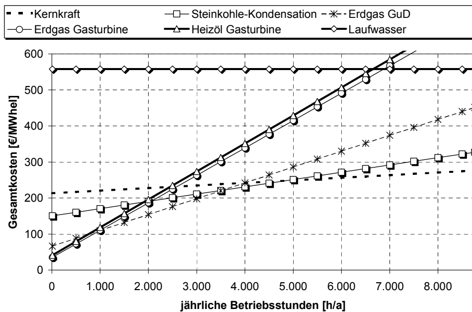
Abb. D-13: Langfristiges Preisgleichgewicht wichtiger zukünftiger Kraftwerkstechnologien in Abhängigkeit der jährlichen Betriebsstunden
