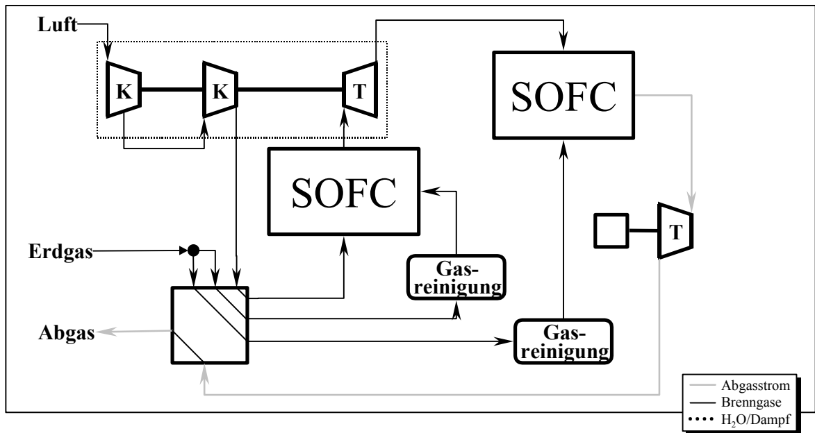
Abb. B-9: Flussschema eines SOFC-Hybridsystems (nachgeschaltete rekuperative Gasturbine)
