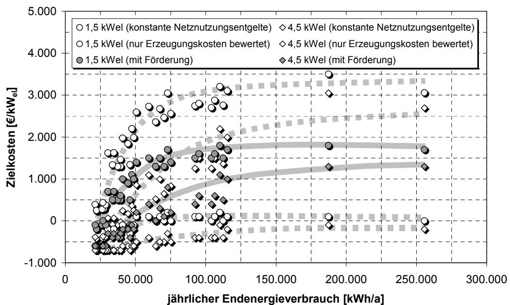
Abb. 4-29: Einfluss einer erzeugungsorientierten Förderung gemäß KWKG auf die Wirtschaftlichkeit von Brennstoffzellen in der Gebäudeversorgung im optimistischen Szenario
