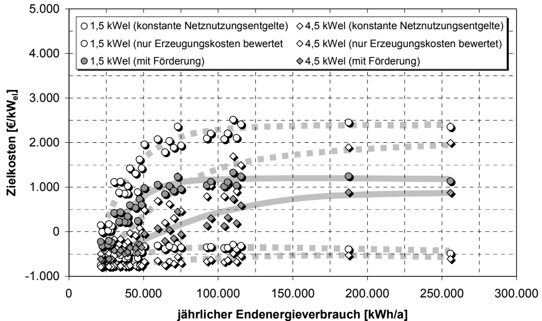
Abb. 4-28: Einfluss einer erzeugungsorientierten Förderung gemäß KWKG auf die Wirtschaftlichkeit von Brennstoffzellen in der Gebäudeversorgung im pessimistischen Szenario
