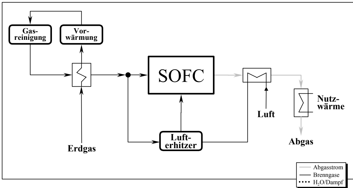
Abb. B-7: Flussschema eines dezentralen KWK-Systems auf Basis der SOFC
