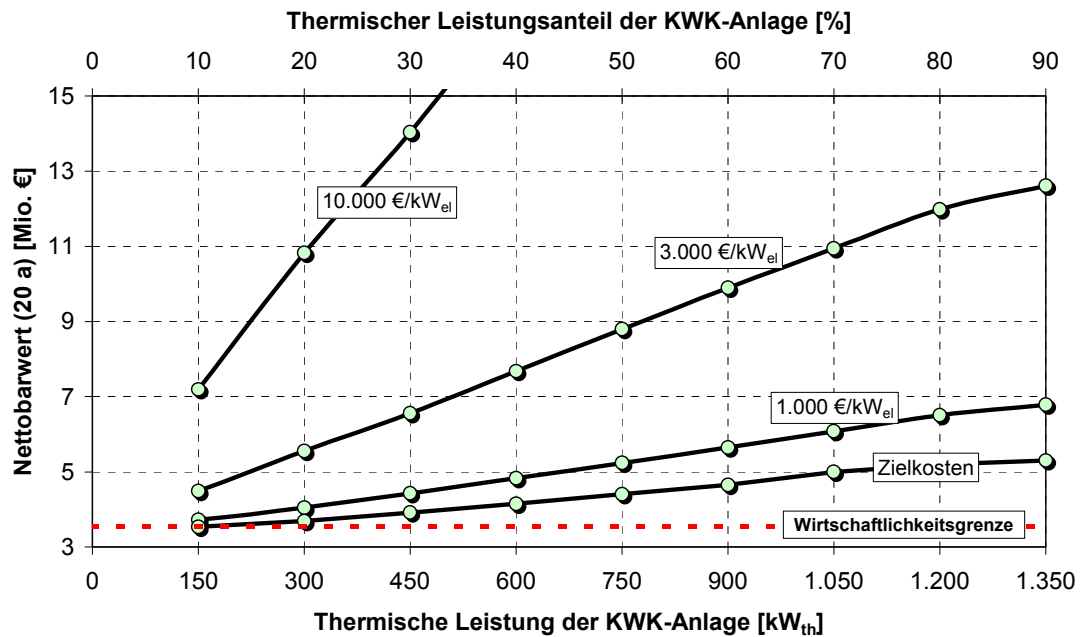
Abb. 4-11: Iterative Zielkostenbestimmung am Beispiel von Hochtemperaturbrennstoffzellen in der chemischen Industrie (50-99 Beschäftigte) im pessimistischen Preisszenario
