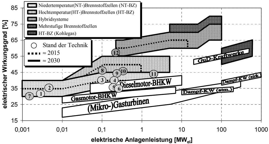
Abb. 2-10: Wirkungsgradvergleich konventioneller Technologien mit stationären Brennstoffzellen in der zeitlichen Perspektive
