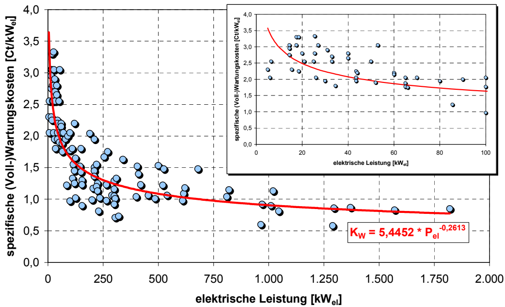
Abb. C-10: Spezifische Wartungskosten gasbetriebener Motor-HKW
