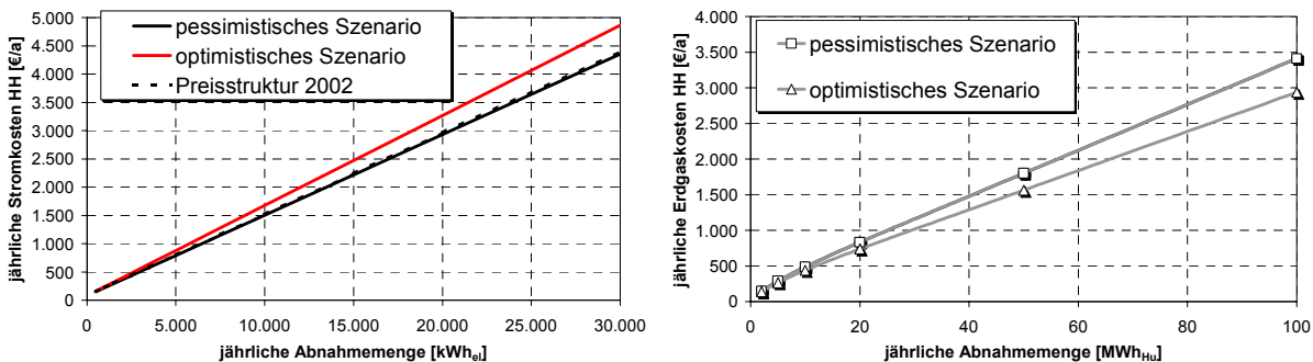
Abb. 4-9: Strom- und Erdgaspreise für ausgewählte Einsatzfälle in den Haushalten Baden-Württembergs im Szenarienvergleich
