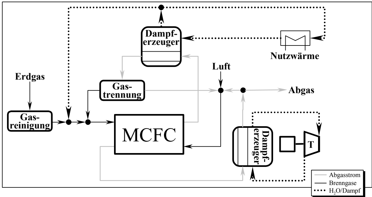
Abb. B-5: Flusschema eines MCFC-Hybridsystems (nachgeschaltete Dampfturbine)
