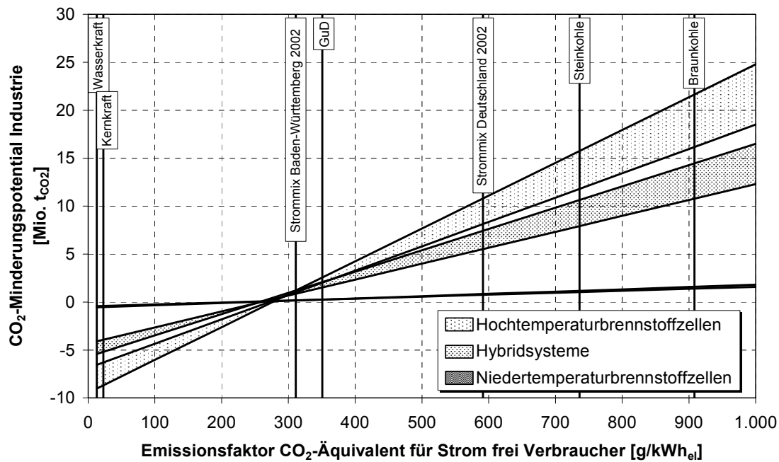
Abb. 4-23: CO 2 -Minderung industrieller Brennstoffzellen in Baden-Württemberg bei spezifischen Investitionskosten von 600 €/kW el und einer günstigen Energiepreisentwicklung in Abhängigkeit von der Emissionsbewertung für Strom
