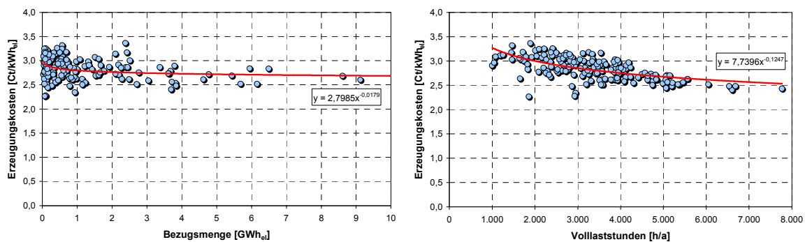
Abb. D-5: Vergleich der berechneten Erzeugungskosten
