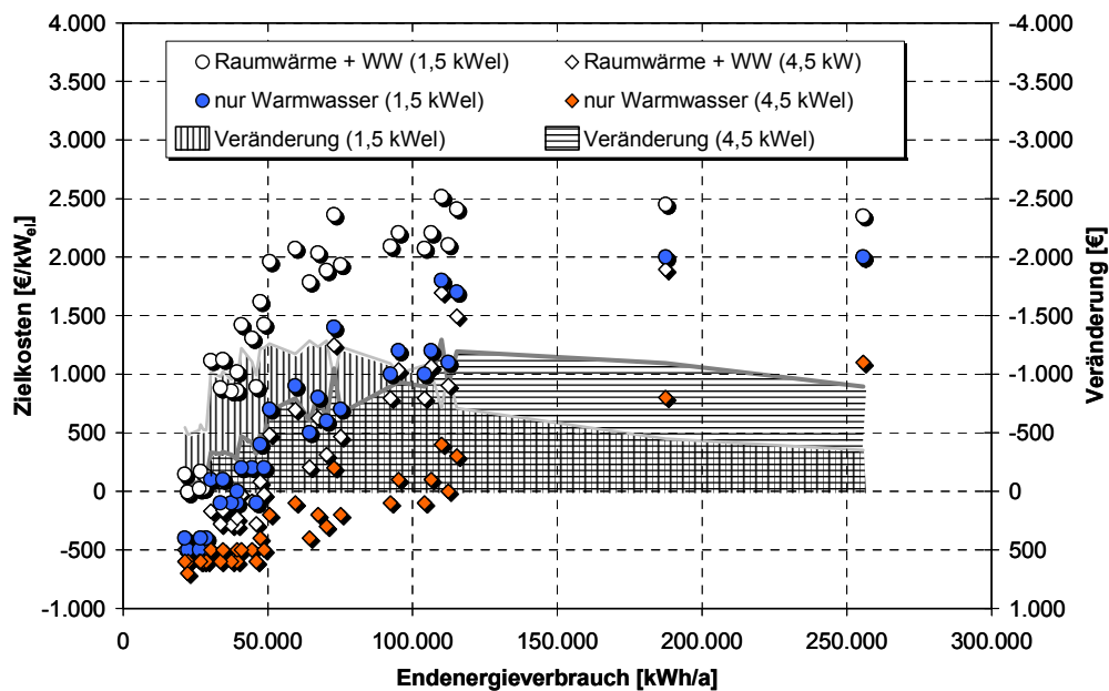
Abb. 4-32: Auswirkungen einer auf die Warmwasserbereitstellung beschränkten Abwärmenutzung (Gebäudebestand) im pessimistischen Preisszenario
