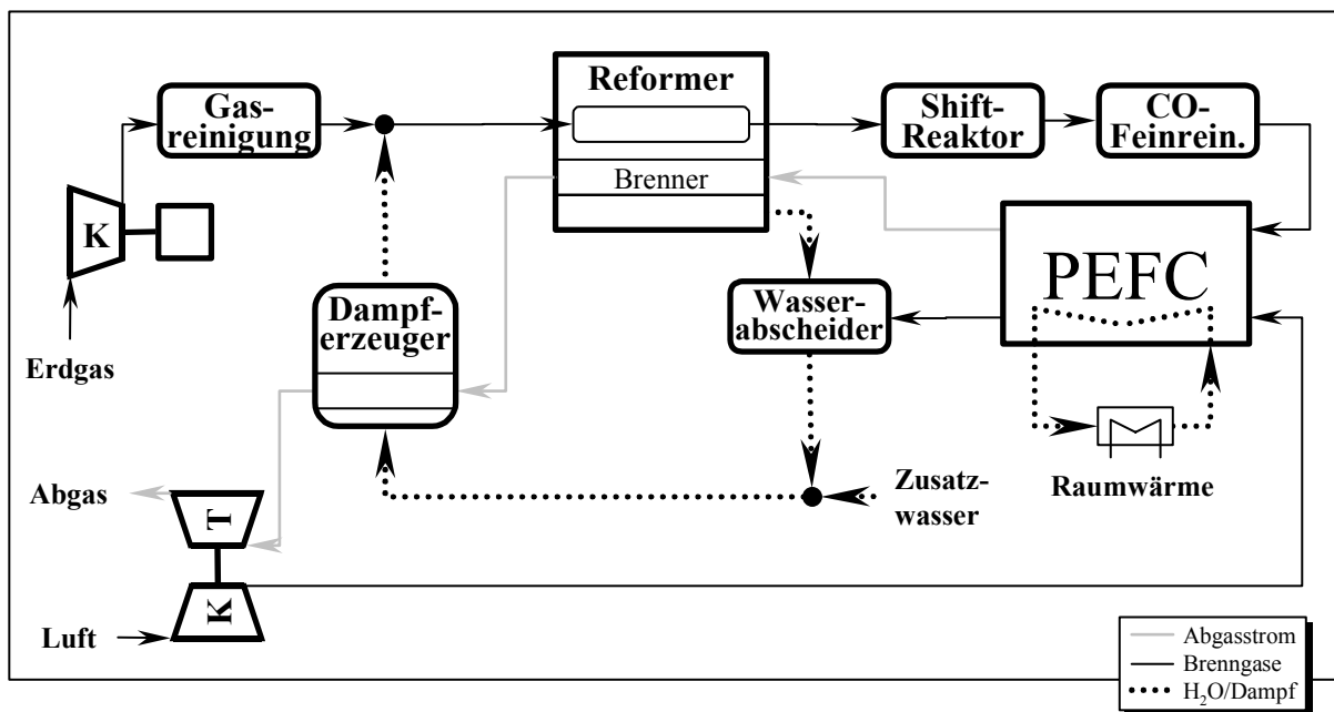
Abb. B-2: Flusschema eines dezentralen KWK-Systems auf Basis der PEFC
