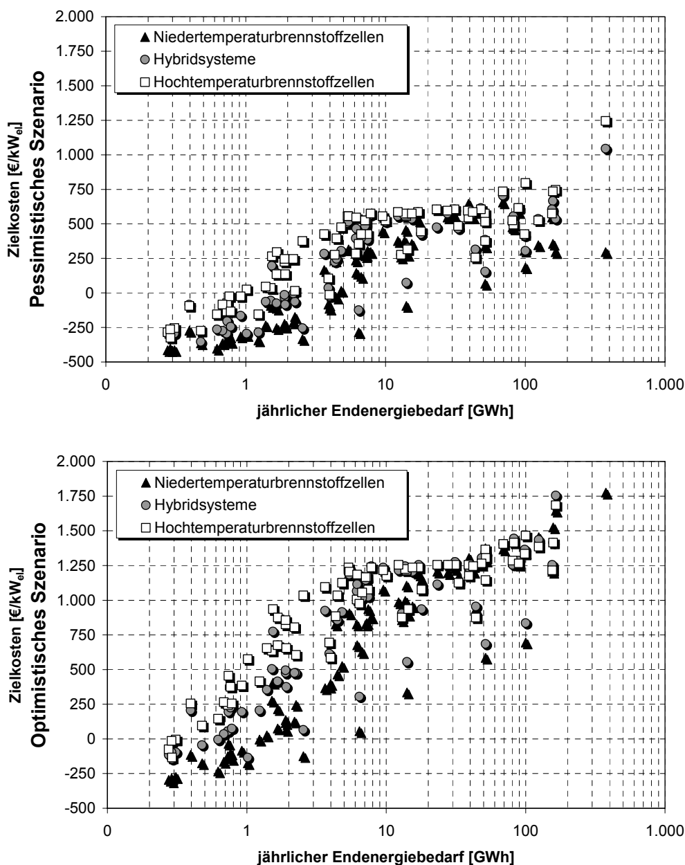
Abb. 4-14: Zu erreichende Zielkosten stationärer Brennstoffzellen im industriellen Sektor
