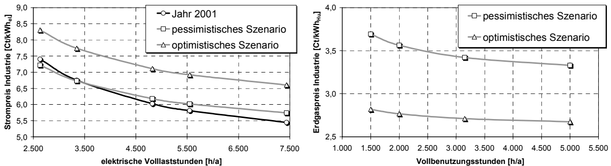
Abb. 4-8: Strom- und Erdgaspreise für ausgewählte Einsatzfälle in der Industrie Baden-Württembergs im Szenarienvergleich
