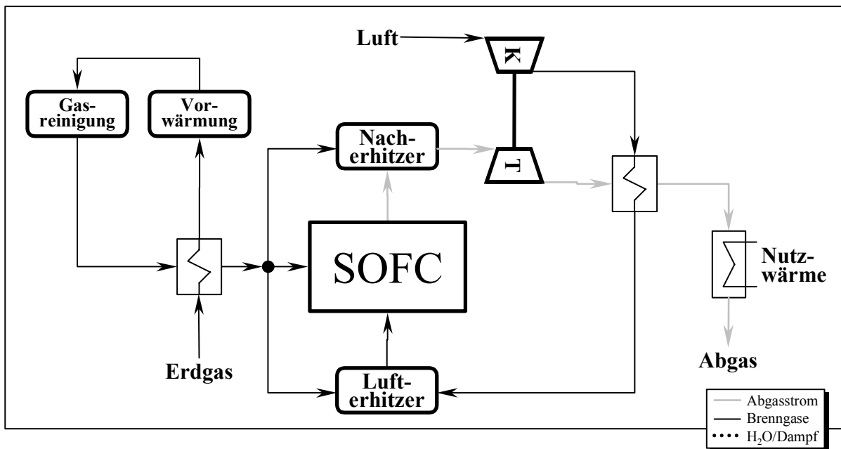
Abb. B-8: Flussschema eines SOFC-Hybridsystems (nachgeschaltete Gasturbine)
