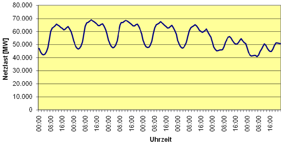
Abbildung 5-1: Netzlustverlauf in Deutschland über einen Zeitraum von einer Woche /UCTE 2009/
