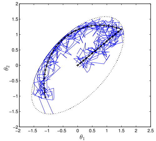
(d) Recursive Constrained ML
