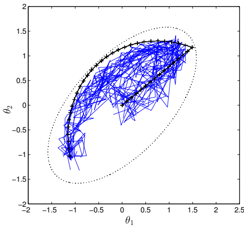
(g) MMSE
