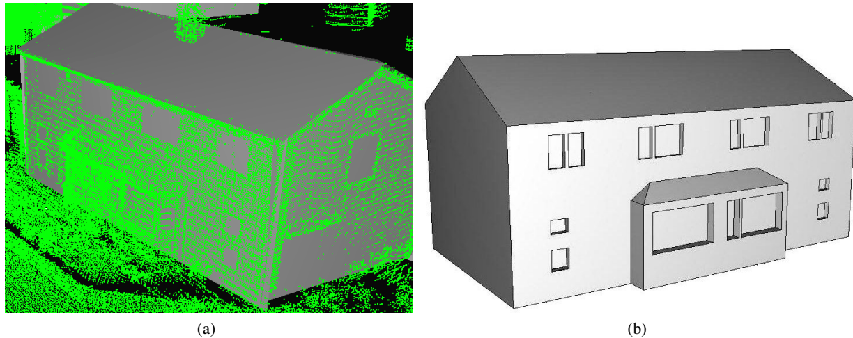
Abbildung 4.12: Datensatz „Red House Farm“: Punktwolke mit grobem Gebäudemodell (a), verfeinertes Gebäudemodell nach rekursiv durchgeführter Fassadenrekonstruktion (b).
