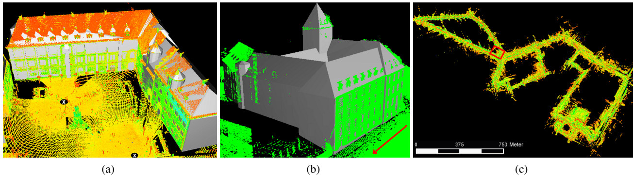
Abbildung 7.1: Typische Aufnahmeconfigurationen für statisches Laserscanning am Beispiel des Schillerplatzes (a) sowie für mobiles Laserscanning am Beispiel des Linden-Museums (b) (Fahrtrichtung durch Pfeil markiert); Übersicht über die mit dem StreetMapper in Stuttgart erfasste Punktwolke (c) (Bereich des Linden-Museums durch Polygon markiert).
