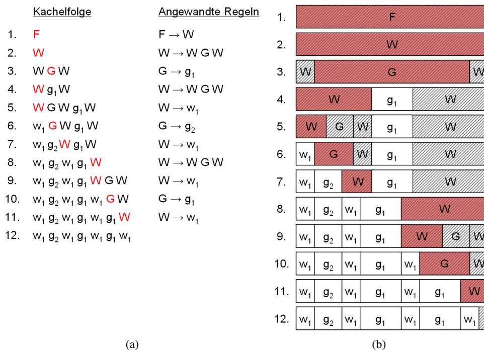
Abbildung 6.1: Nichtterminal-Selektion.
