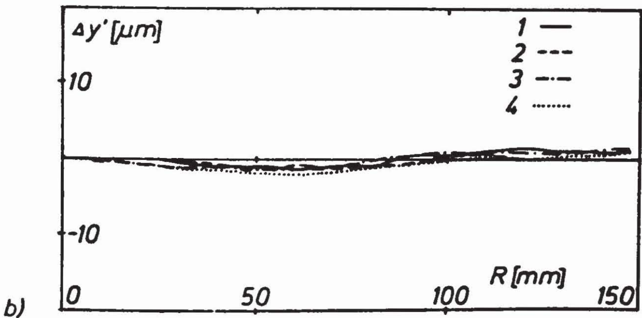
Abb. 1: Ergebnisse der Verzeichnungsmessung eines Luftbildobjektives der neuen Generation der Brennweite f' = 152,8 \text{ mm} und der Blende F/4 a) für eine Bildhalbdiaagonale b) für vier Bildhalbdiaagonalen
