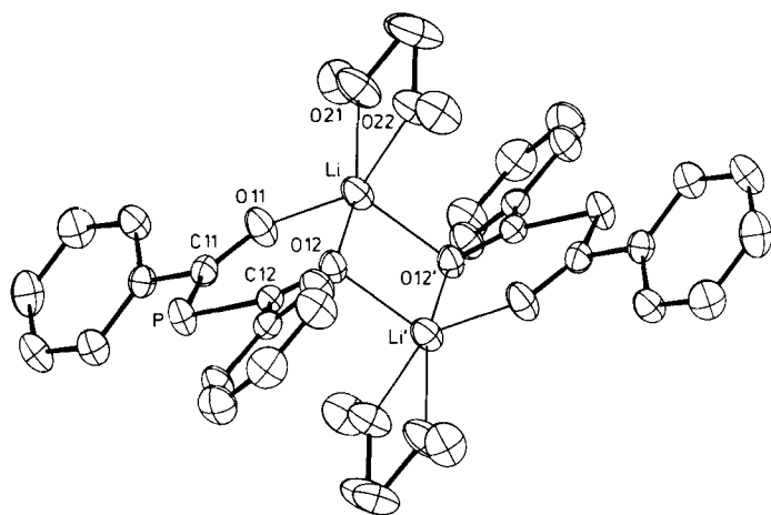
Abb. 1. ORTEP-Zeichnung der Molekülstruktur von dimerem Lithiumdibenzoylphosphid·1,2-Dimethoxyethan. Die Schwingungsellipsoide entsprechen einer Aufenthaltswahrscheinlichkeit von 50%. (2), Raumgruppe P2_1/c , a = 1907.1(7) , b = 762.6(7) , c = 1259(2) pm; \beta = 104.5(1)^\circ ; 4 Formeleinheiten. 1907 unabhängige, beobachtete ( F > \sigma ) Reflexe wurden auf einem automatischen Vierkreisdiffraktometer CAD4 (Enraf-Nonius) bei -80^\circ\text{C} gemessen ( \text{MoK}\alpha -Strahlung, 4^\circ < 2\theta < 48^\circ ) und in üblicher Weise korrigiert; R_w = 0.034 .
