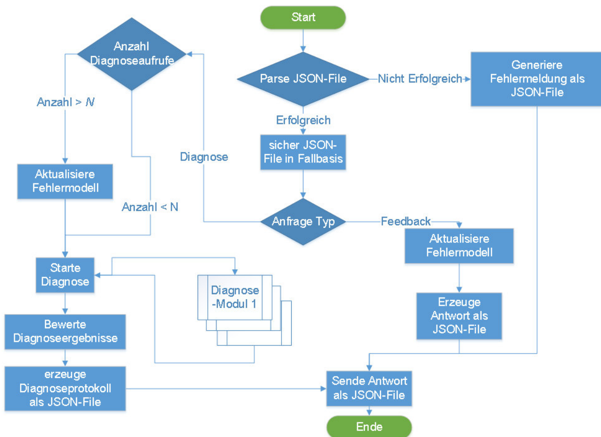
Abbildung 3.16: Systemablaufdiagramm
