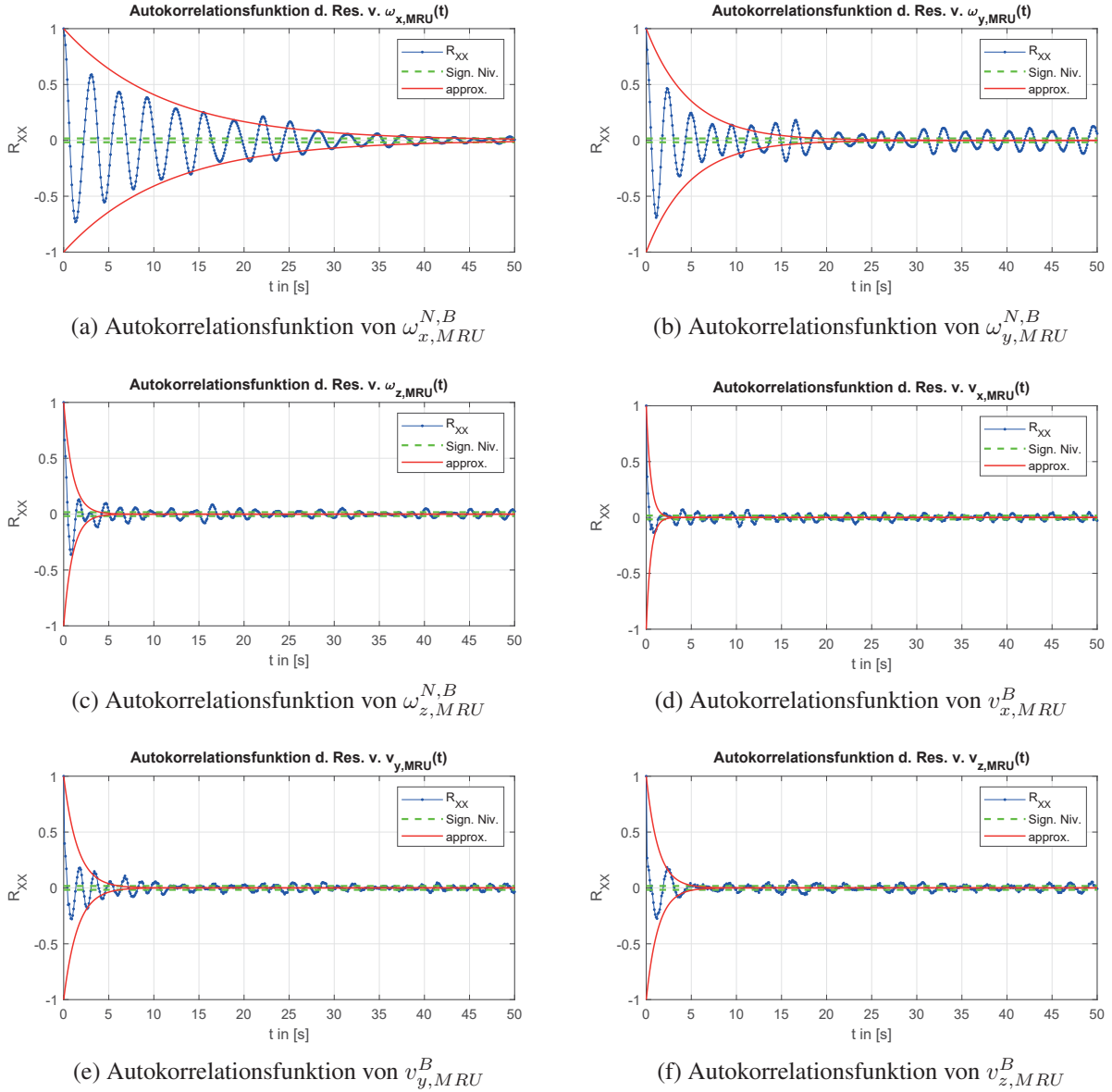
Abb. 3.20: Exemplarische Ausschnitte der Autokorrelationsfunktionen
