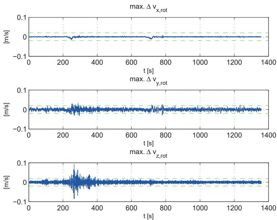
Abb. 5.5: Einfluss von \Delta \mathbf{v}_{Rot}^B auf \bar{\mathbf{v}}_{k+1}^B für \Delta \mathbf{p}_{CG}^B = [15, 48 \text{ m } 3, 87 \text{ m } 1 \text{ m}]^T im Vergleich zur Messgenauigkeit (grüne Linie)
