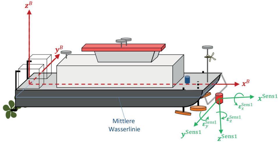
Abb. 2.3: Schiffskoordinatensystem \mathbf{x}^B und Sensorkoordinatensystem \mathbf{x}^{\text{Sens}} (von einem Sensor)
