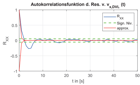
Abb. A.10: Ausschnitt aus der Autokorrelationsfunktion v_{x,DVL} (ohne determ. Anteil)
