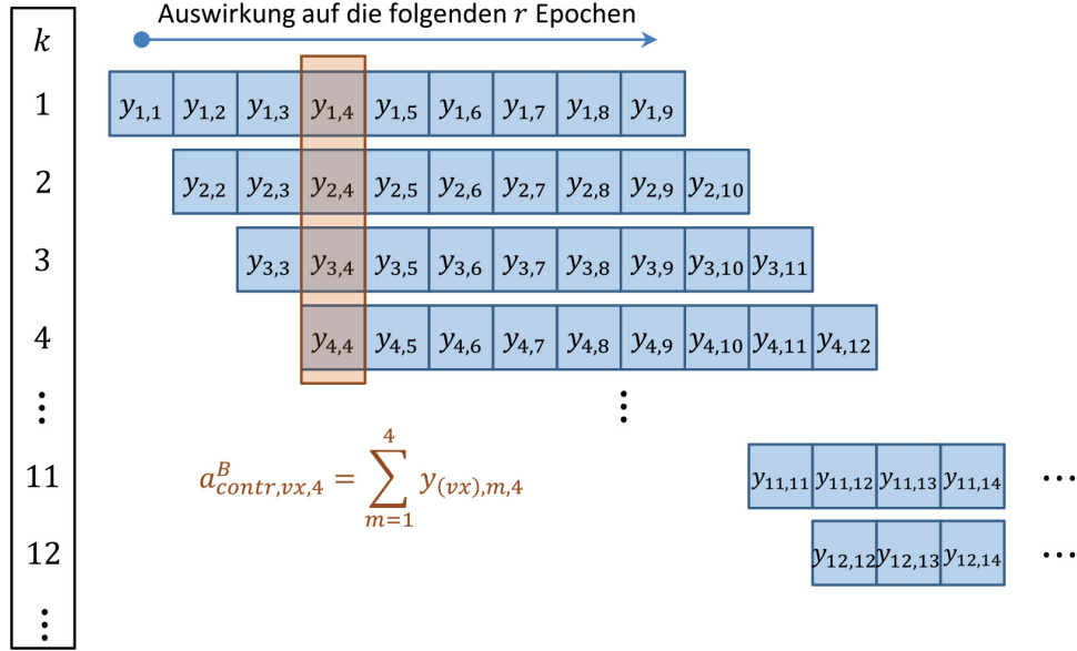
Abb. 4.5: Bestimmung der bei t_k wirksamen Beschleunigung a_k^B bei einer Regelstrecke der Länge r - hier exemplarisch für a_4 ( k = 4 ) und h = v_x dargestellt.
