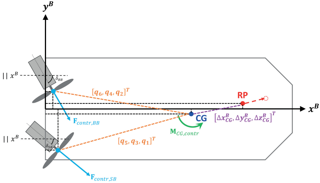
Abb. 4.3: Einfluss eines am Massenschwerpunkt CG wirkenden Drehmoments M_{CG,contr} , resultierend aus den Kraftvektoren F_{contr,SB} und F_{contr,BB} (zwei Propeller), auf das Bewegungsverhalten am Referenzpunkt RP
