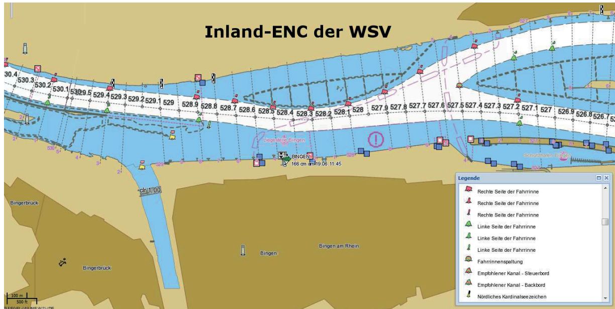
Abb. 1.1: Inland-ENC der WSV - Elektronische Navigationskarte entsprechend dem internationalen ECIDS-Standard, Rhein bei Bingen, WSV (2017)
