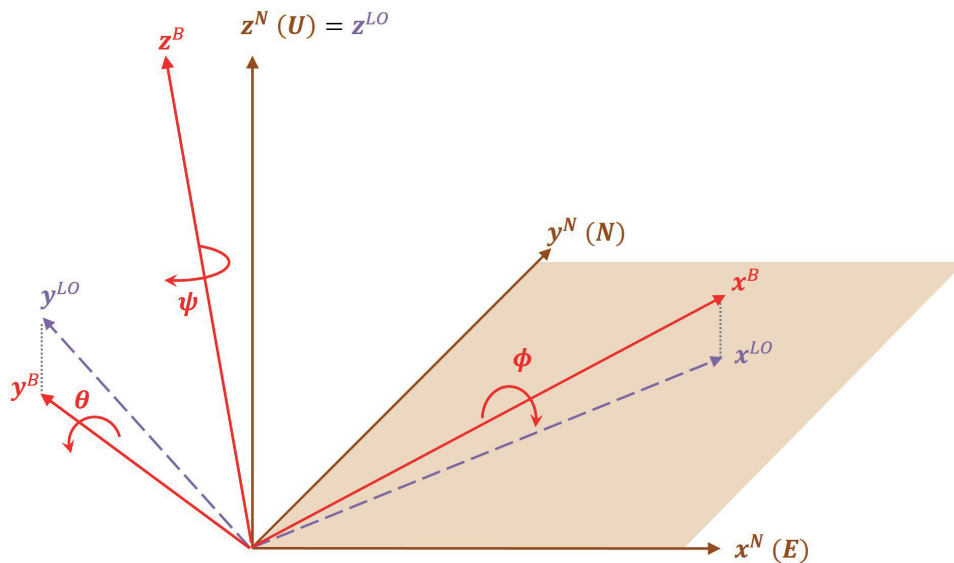
Abb. 2.4: Navigationskoordinatensystem \mathbf{x}^N , projiziertes Schiffskoordinatensystem \mathbf{x}^{LO} und Schiffskoordinatensystem \mathbf{x}^B
