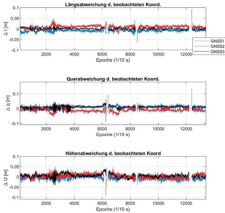
Abb. 5.10: Innovationen-basierte Längs- und Querabweichungen und d_{U,GNSS,k+1} bei Anwendung der regionalen VKS nur für \sigma_{w,\omega}^2 (Modellerweiterung KINEMATIK, Szenario 3)
