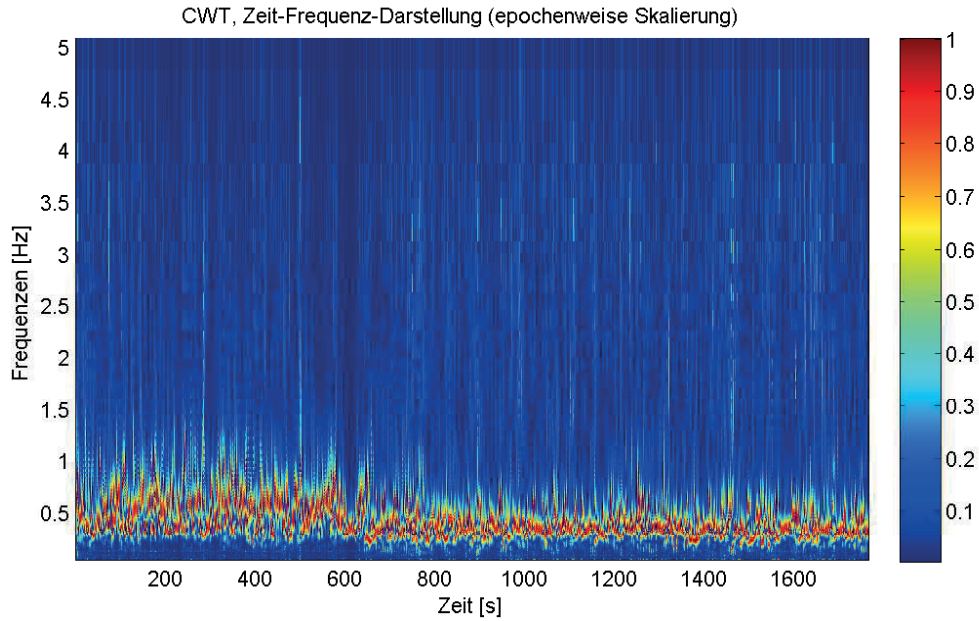
Abb. 3.23: Zeit-Frequenzdarstellung der CWT (epochenweise Skalierung) für \Delta\omega_{x,MRU}^{B,N}
