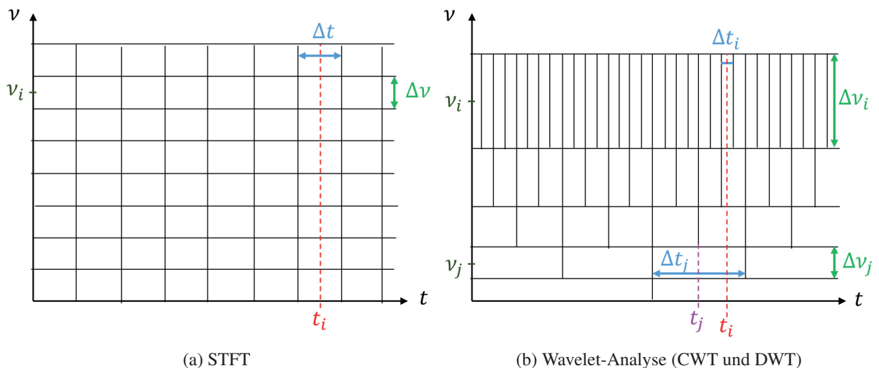
Abb. 3.14: Zeitliche und spektrale Auflösung bei der Signalanalyse mit Fourier-Transformation und Wavelet-Analyse
