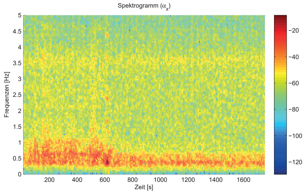
Abb. 3.24: Spektrogramm (Power Spectral Density) für \Delta\omega_{x,MRU}^{B,N}
