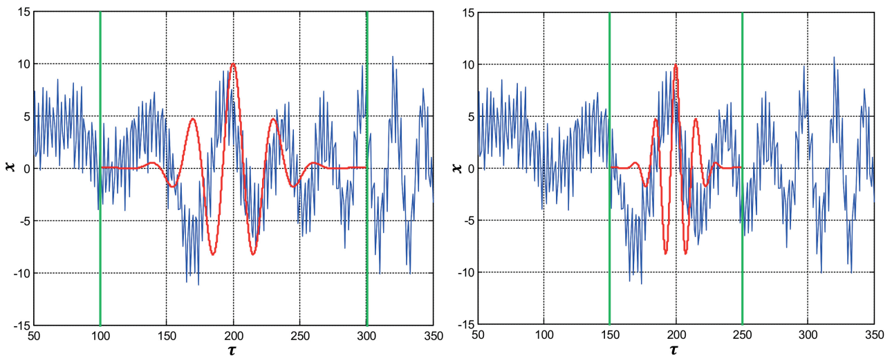
Abb. 3.6: Ein Wavelet (rot) mit unterschiedlichen Skalierungen wird über das Signal (blau) verschoben; Analyse des grün markierten Signalbereichs
