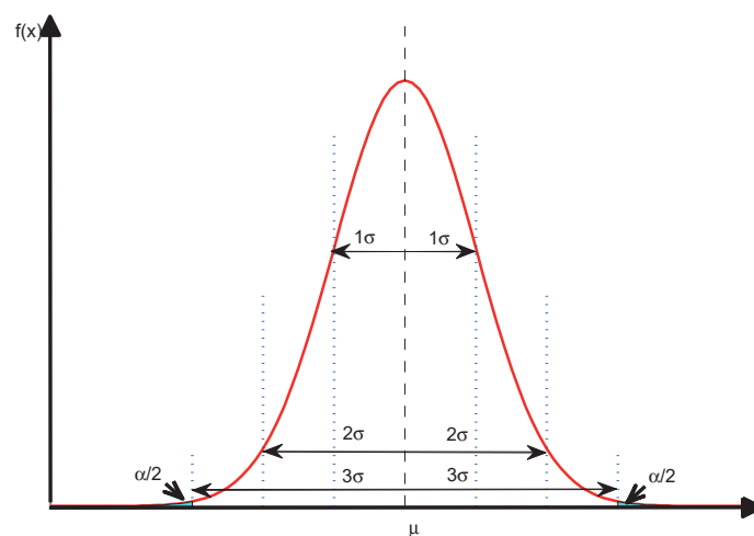
Abb. 3.15: Normalverteilung mit den Vertrauensintervallen
