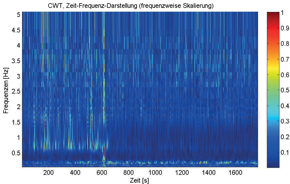
Abb. 3.22: Zeit-Frequenzdarstellung der CWT (frequenzweise Skalierung) für \Delta\omega_{x,MRU}^{B,N}
