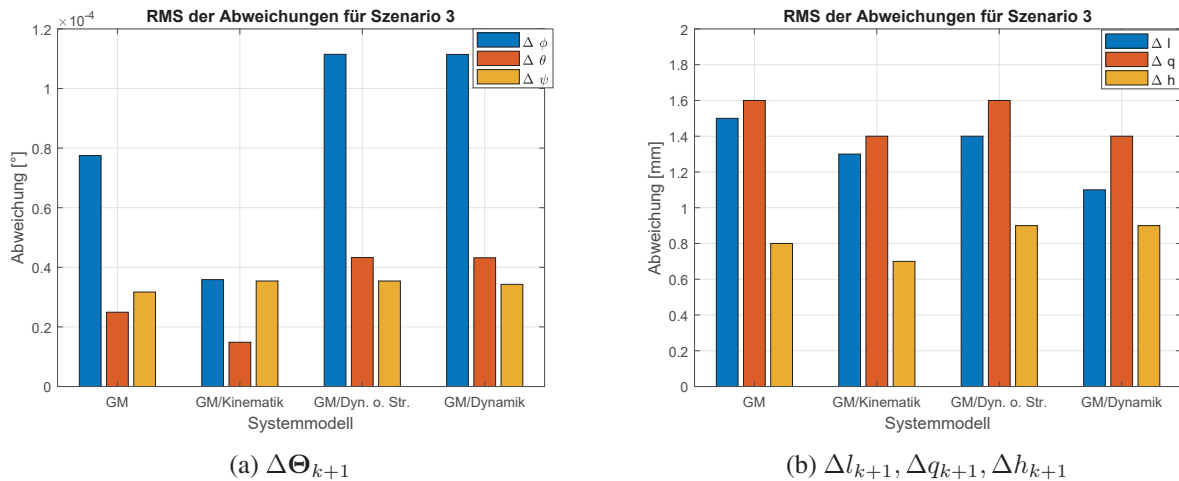
Abb. 5.17: Abweichungen zwischen geschätzten und prädierten Größen in Szenario 3 bei Verwendung der unterschiedlichen Systemmodellen
