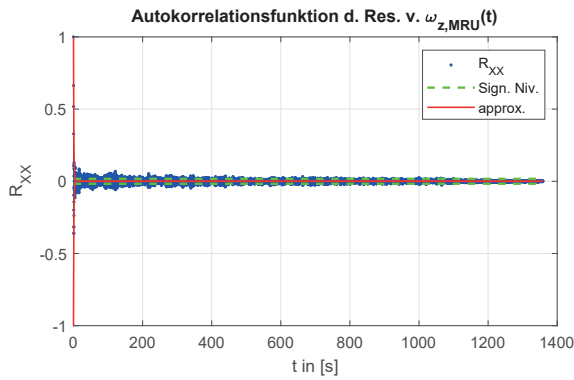
Abb. A.3: Autokorrelationsfunktion \omega_{z,MRU} (ohne determ. Anteil)
