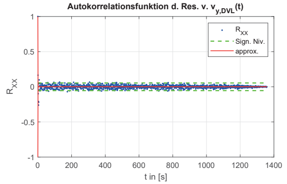
Abb. A.8: Autokorrelationsfunktion v_{y,DVL} (ohne determ. Anteil)
