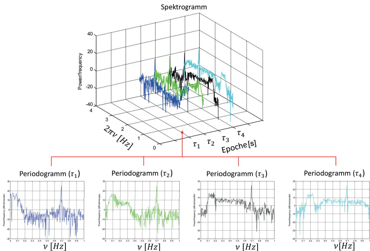
Abb. 3.4: Darstellung des Ergebnisses einer STFT: Aufbau eines Spektrogramms aus Periodogrammen für die jeweilige Verschiebungsparameter \tau^\gamma = [\tau_1, \tau_2, \tau_3, \tau_4] (spektrale Leistungsdichte / PSD)
