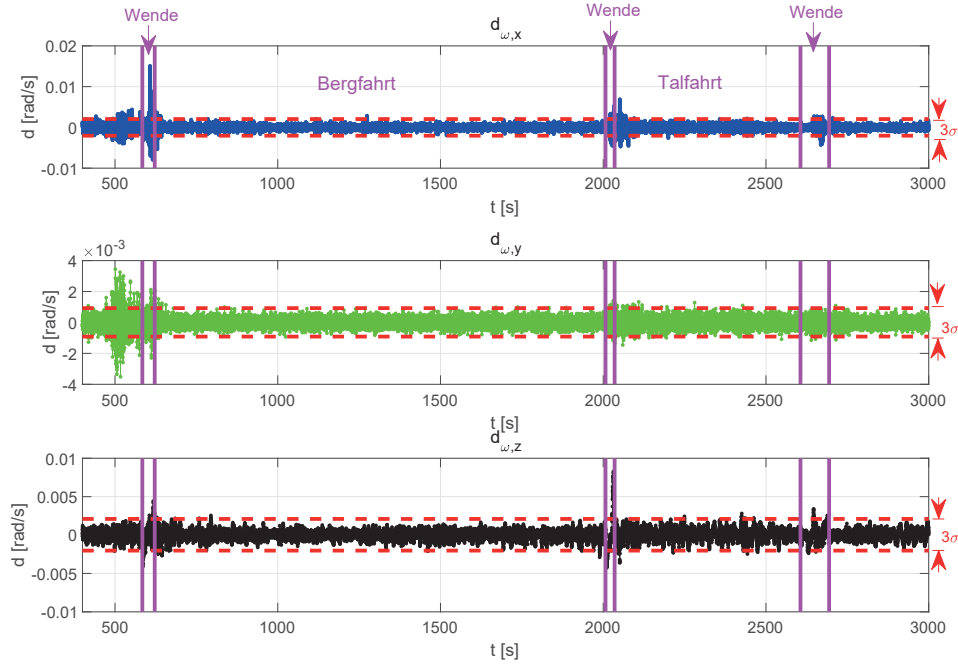
Abb. 5.12: Modellerweiterung DYNAMIK/Antrieb und zyklische Effekte: Innovationen der Drehraten ( d_{\omega,x,MRU,k+1} , d_{\omega,y,MRU,k+1} , d_{\omega,z,MRU,k+1} ) in verschiedenen Fahrtabschnitten für Szenario 2 im Vergleich zu \pm 3\sigma_d (rote Linien)
