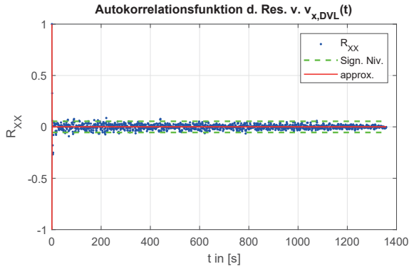
Abb. A.7: Autokorrelationsfunktion v_{x,DVL} (ohne determ. Anteil)
