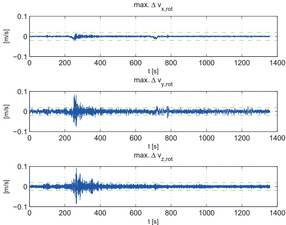
Abb. 5.4: Einfluss von \Delta \mathbf{v}_{rot}^B auf \bar{\mathbf{v}}_{k+1}^B für \Delta \mathbf{p}_{CG}^B = [15, 48 \text{ m } 3, 87 \text{ m } 4, 56 \text{ m}]^T im Vergleich zur Messgenauigkeit (grüne Linie)
