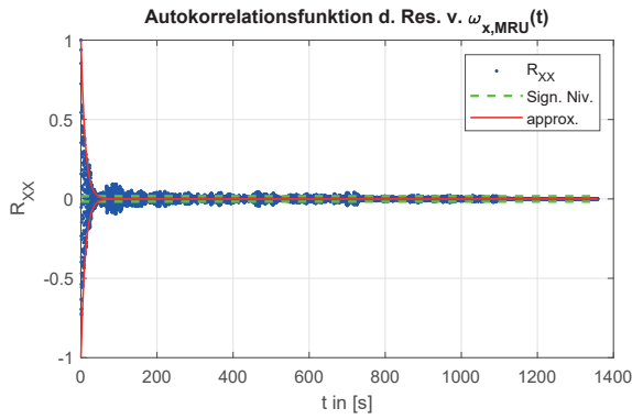
Abb. A.1: Autokorrelationsfunktion \omega_{x,MRU} (ohne determ. Anteil)
