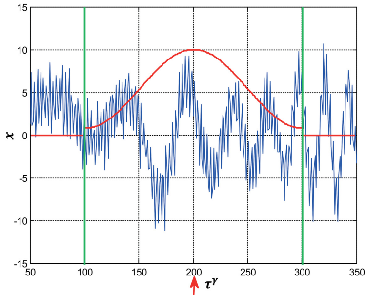
Abb. 3.3: Fensterung eines Signals mit der Fensterfunktion des Hamming-Fensters (rot), die dem Zeitpunkt \tau^\gamma = 200 s zugeordnet ist
