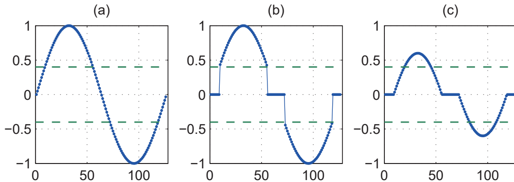
Abb. 3.18: Rauschminderung am Beispiel des (a) Signals x(t) mit (b) hard Thresholding und (c) soft Thresholding , nach Misiti et al. (2007)
