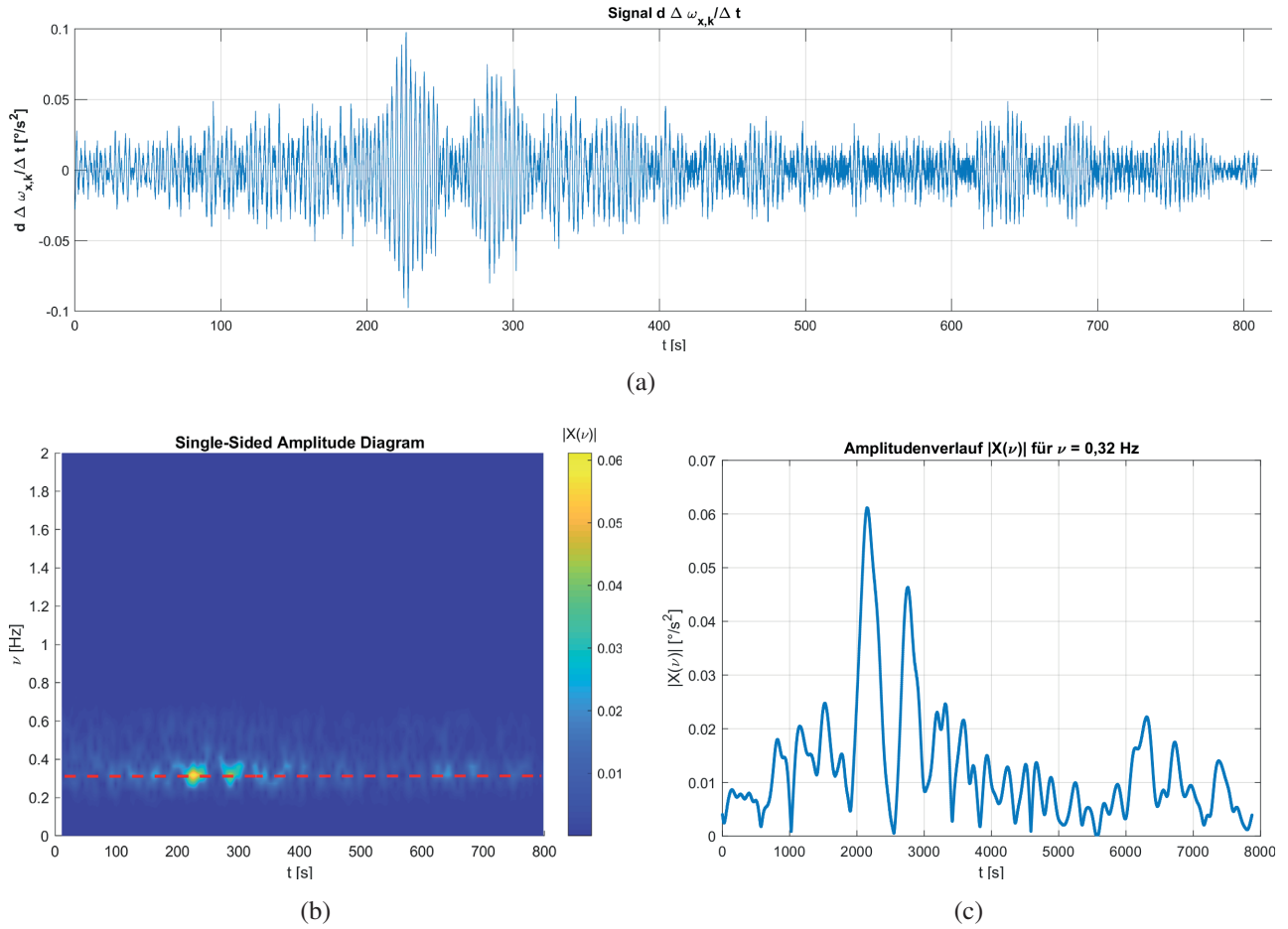
Abb. 3.27: Exemplarische Analyse des (a) verbleibenden Anteils von \Delta \omega_{x,k}/\Delta t mittels (b) STFT (hier Darstellung als Amplitudendiagramm) und (c) Darstellung des variierenden Amplitudenverlaufs für \nu = 0,32 Hz (Rote Linie in (b))
