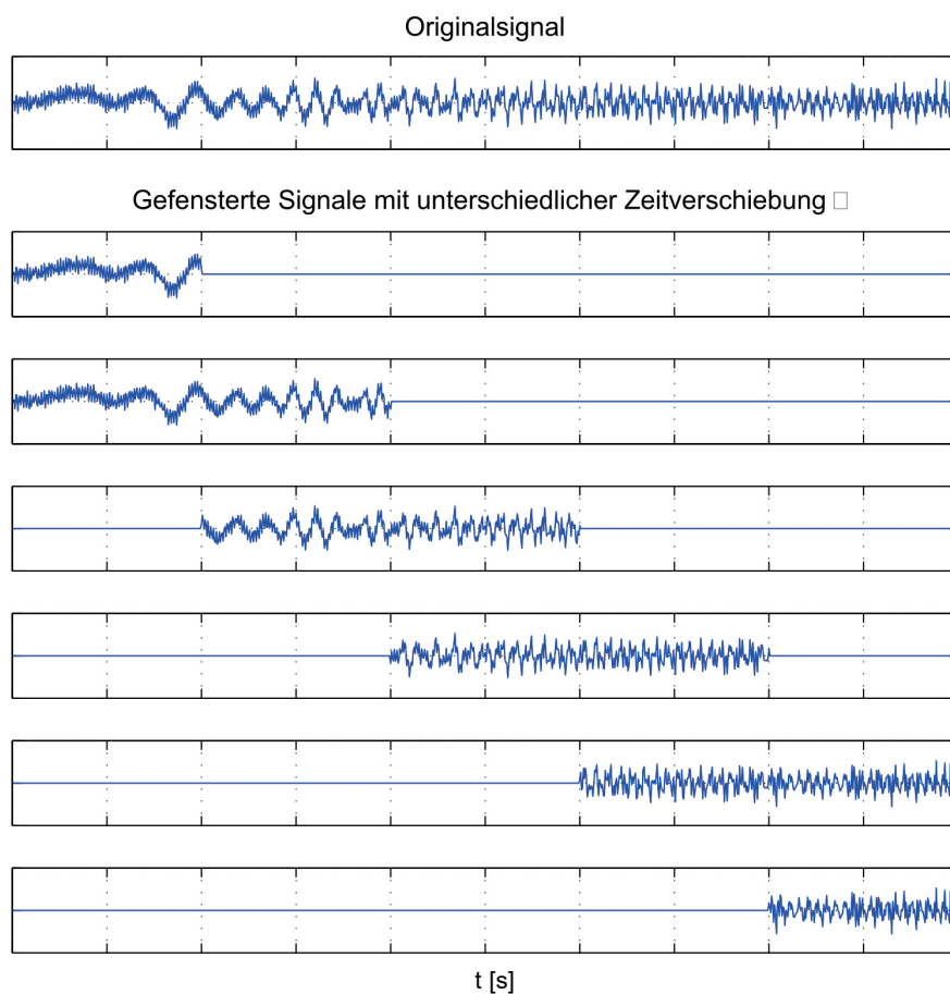
Abb. 3.1: Fensterung eines Signals mit einem Rechteckfenster (MATLAB, Beispieldatensatz noismima )
