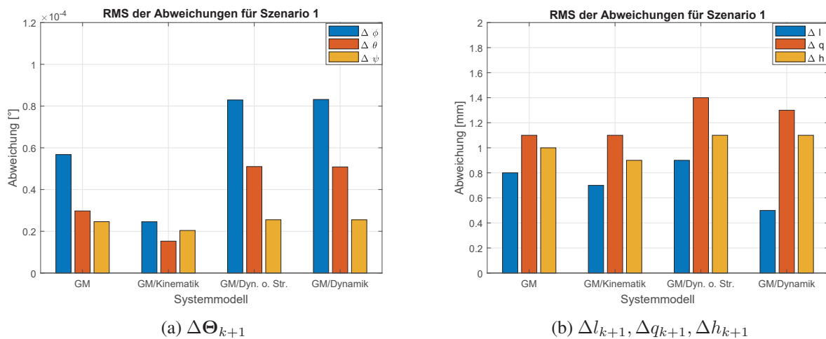
Abb. 5.15: Abweichungen zwischen geschätzten und prädizierten Größen in Szenario 1 bei Verwendung der unterschiedlichen Systemmodellen
