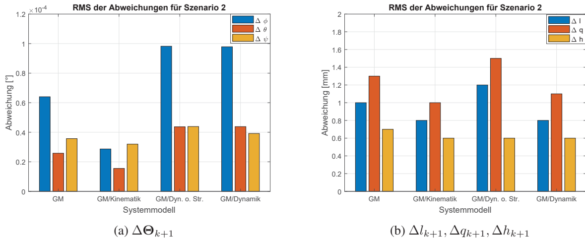
Abb. 5.16: Abweichungen zwischen geschätzten und prädierten Größen in Szenario 2 bei Verwendung der unterschiedlichen Systemmodellen
