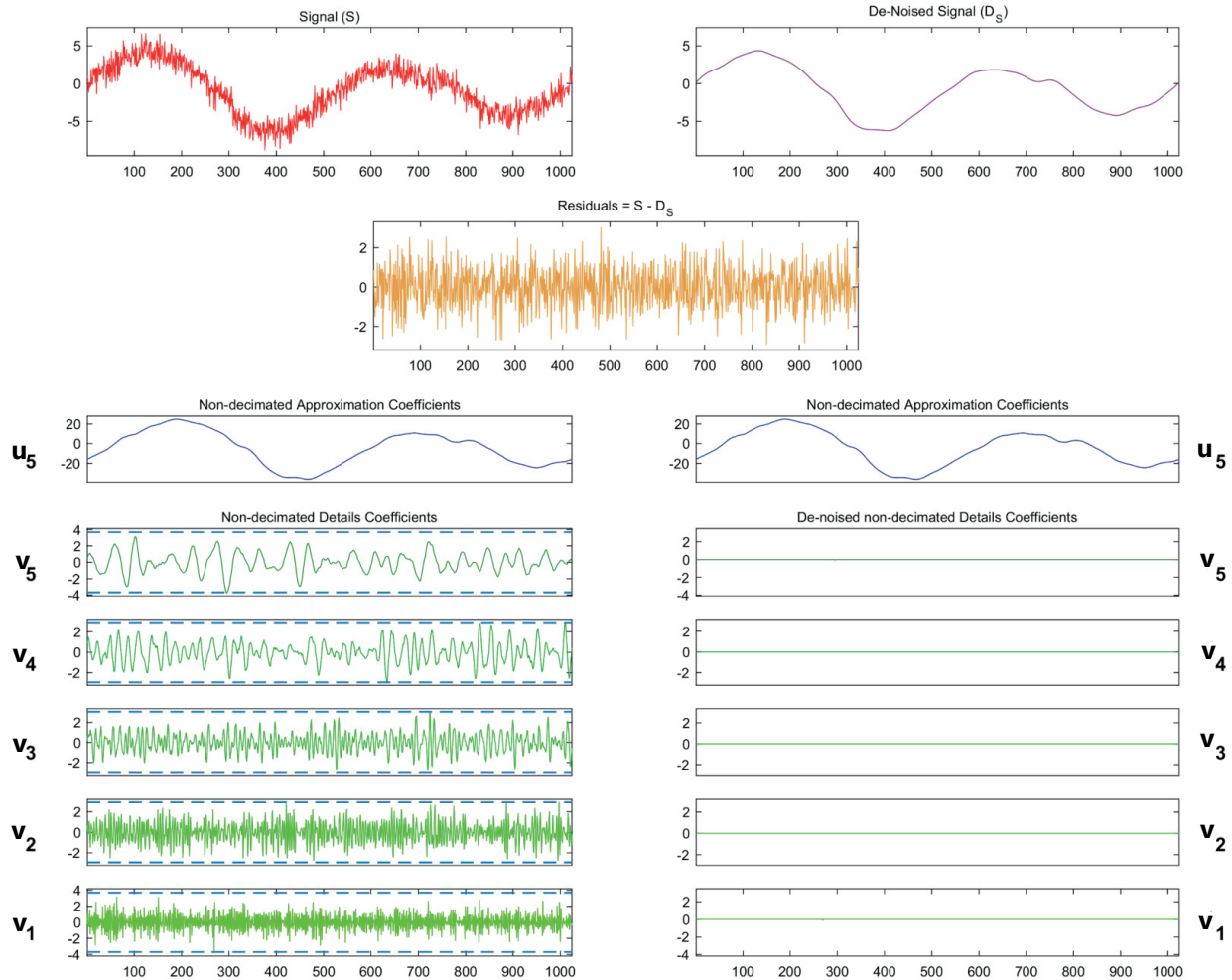
Abb. 3.19: Rauschminderung für ein exemplarisches Signal ( heavysin , MATLAB R2018a) in MATLAB mit db4-Wavelet, m = 5 - Zerlegung des Signals S in einen geglätteten Signalanteil D_S und die Residuen
