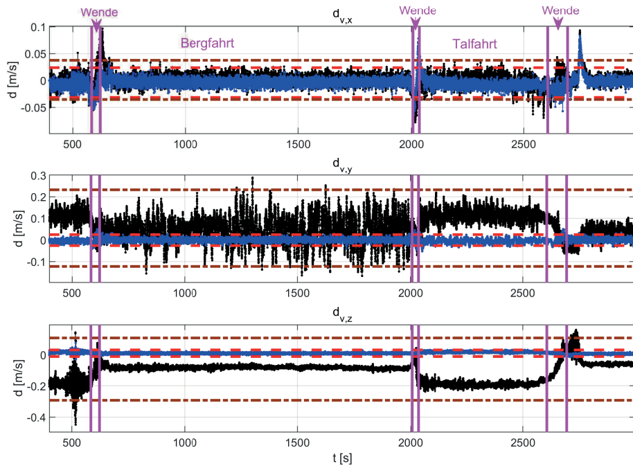
Abb. 5.13: Modellerweiterung DYNAMIK/Antrieb und zyklische Effekte: Innovationen der Geschwindigkeiten ( d_{v,x,MRU,k+1} , d_{v,y,MRU,k+1} , d_{v,z,MRU,k+1} ) in verschiedenen Fahrtabschnitten für Szenario 2 (blau: MRU, schwarz: DVL) im Vergleich zu \pm 3\sigma_d (rote bzw. braune Linien)
