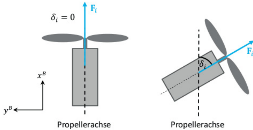
Abb. 4.2: Zugrichtung \delta des Ruderpropellers (Breitenfeld et al. 2015)
