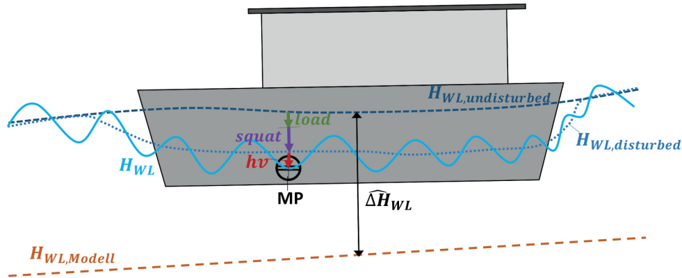
Abb. 4.7: Zusammenhang zwischen der Wasserspiegellage H_{WL} (hydrologisches Modell) und einem Bezugspunkt MP am Schiff (nach Breitenfeld et al. 2015)
