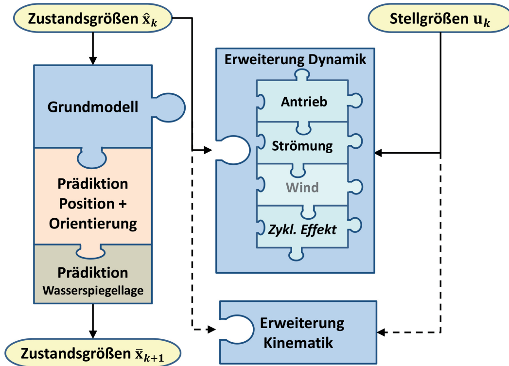
Abb. 4.1: Prädiktionsmodell mit fakultativen Erweiterungen
