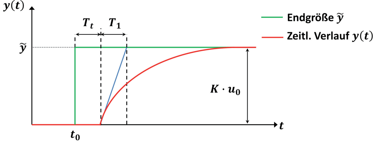
Abb. 4.4: Übertragungsverhalten für eine Größe y(t) aufgrund des PT_1 T_t -Übertragungsglieds
