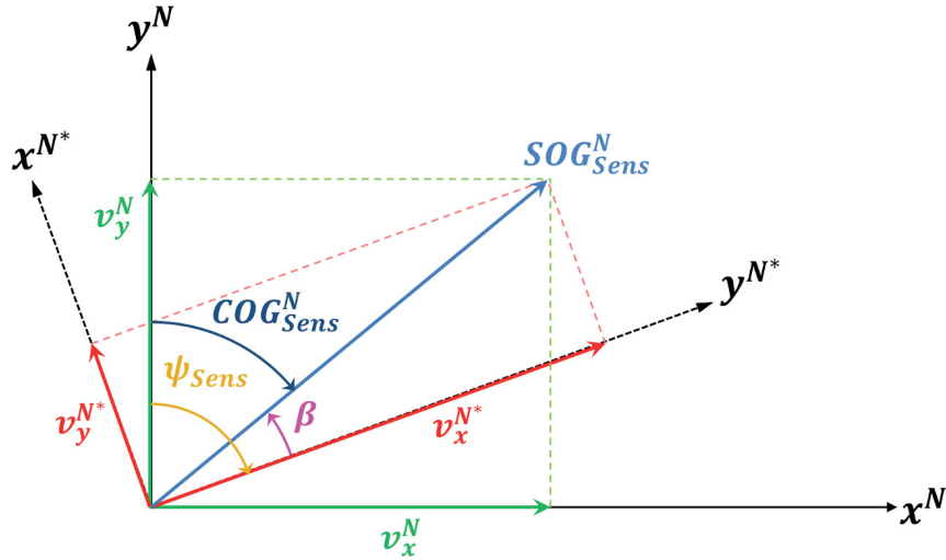
Abb. 4.6: Zusammenhang von SOG_{Sens}^N , COG_{Sens}^N und den verwendeten Koordinatensystemen (Breitenfeld et al. 2015)
