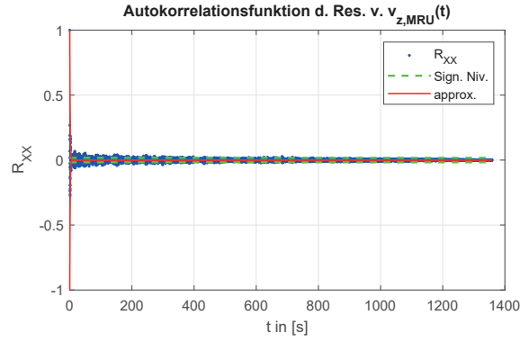
Abb. A.6: Autokorrelationsfunktion v_{z,MRU} (ohne determ. Anteil)
