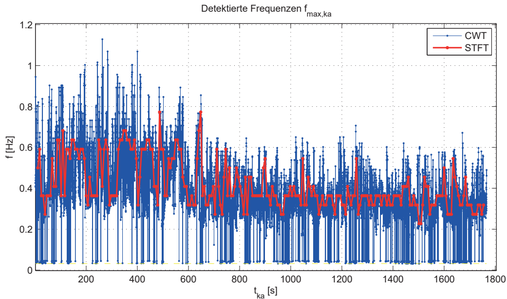
Abb. 3.26: Detektierte dominierende Frequenzen für \Delta\omega_{x,MRU}^{B,N} (0,1 Hz - 1 Hz)
