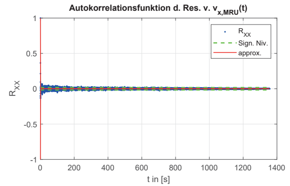
Abb. A.4: Autokorrelationsfunktion v_{x,MRU} (ohne determ. Anteil)
