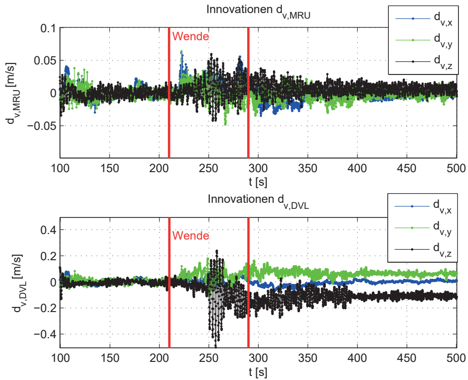
Abb. 5.7: Innovationen bzgl. \mathbf{l}_{v,MRU,k+1} und \mathbf{l}_{v,DVL,k+1} mit auftauchendem Offset
