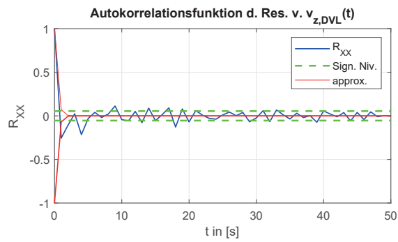
Abb. A.12: Ausschnitt aus der Autokorrelationsfunktion v_{z,DVL} (ohne determ. Anteil)
