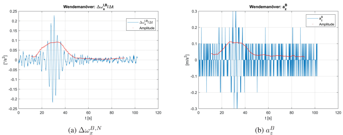
Abb. 3.28: Vergleich: Verbleibender Signalanteil und geschätzte Amplitude für die dominierende Frequenz bei einem exemplarischen Wendemanöver auf dem Rhein (Abschnitt von Fahrt 3)
