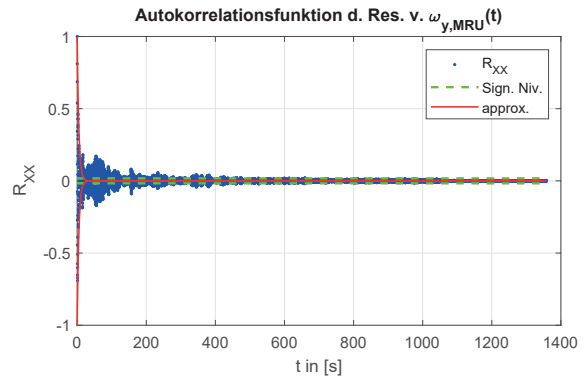
Abb. A.2: Autokorrelationsfunktion \omega_{y,MRU} (ohne determ. Anteil)
