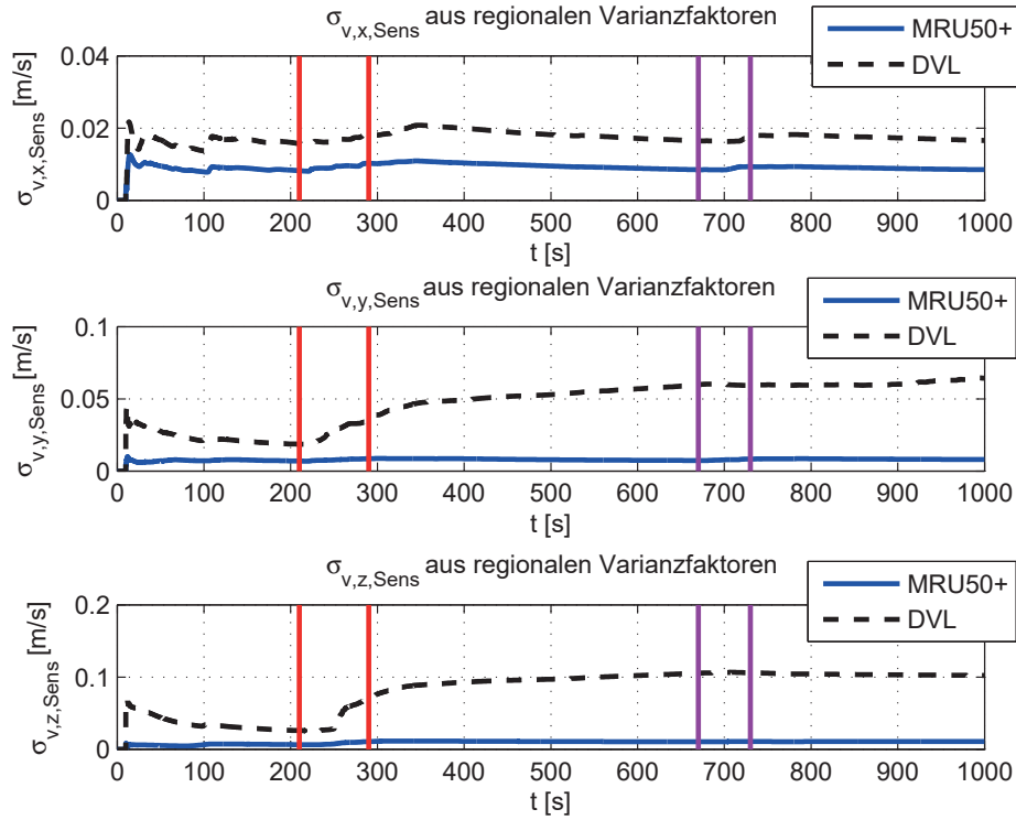
Abb. 5.8: Geschätzte regionale Varianzkomponenten für l_{v,MRU,k+1} und l_{v,DVL,k+1} bei einer Messfahrt mit zwei Wendungen
