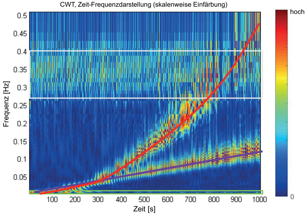
Abb. 3.9: Übertragung des Skalogramms in eine Zeit-Frequenzdarstellung
