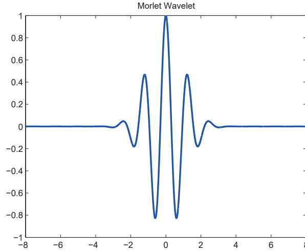
Abb. 3.11: Morlet-Wavelet nach (3.65) (MATLAB)
