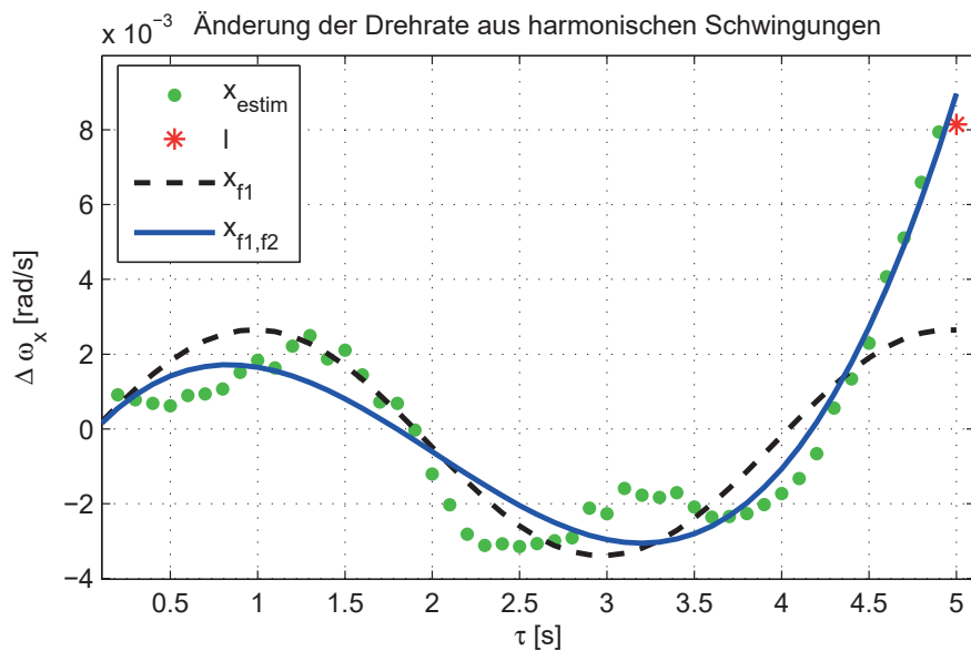
Abb. 5.11: Modellierung der Drehratenänderung \Delta \omega_x durch einen trigonometrischen Polynomterm (schwarz) und durch zwei überlagerte trigonometrische Polynomterme (blau)
