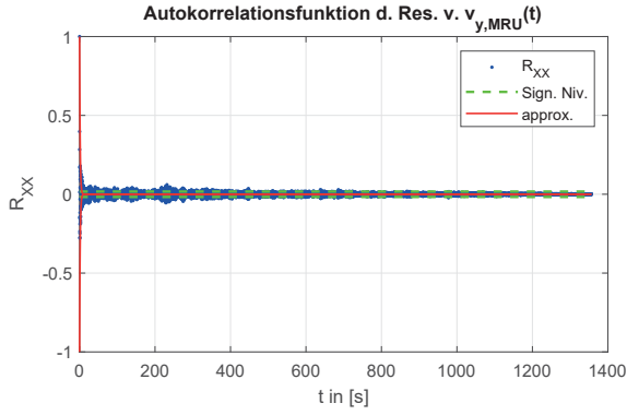
Abb. A.5: Autokorrelationsfunktion v_{y,MRU} (ohne determ. Anteil)
