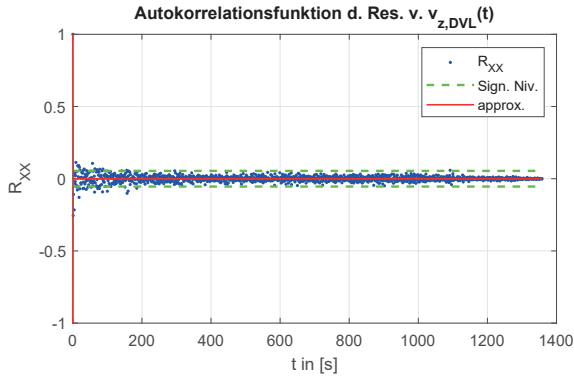
Abb. A.9: Autokorrelationsfunktion v_{z,DVL} (ohne determ. Anteil)
