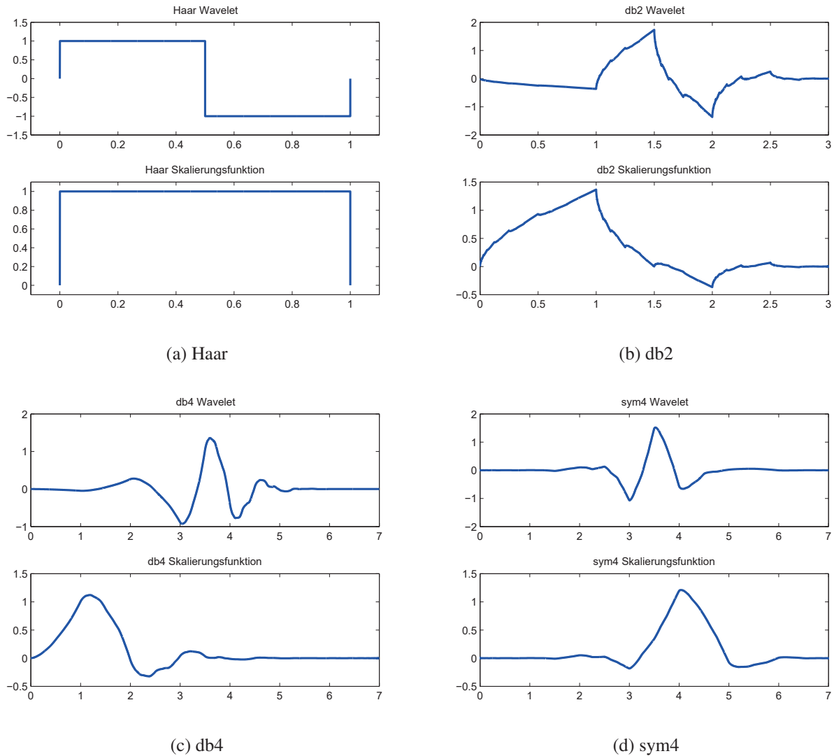
Abb. 3.12: Wavelets und Skalierungsfunktionen: Daubechies-Wavelets (a-c) und Symlet (d) der Ordnung N (MATLAB)
