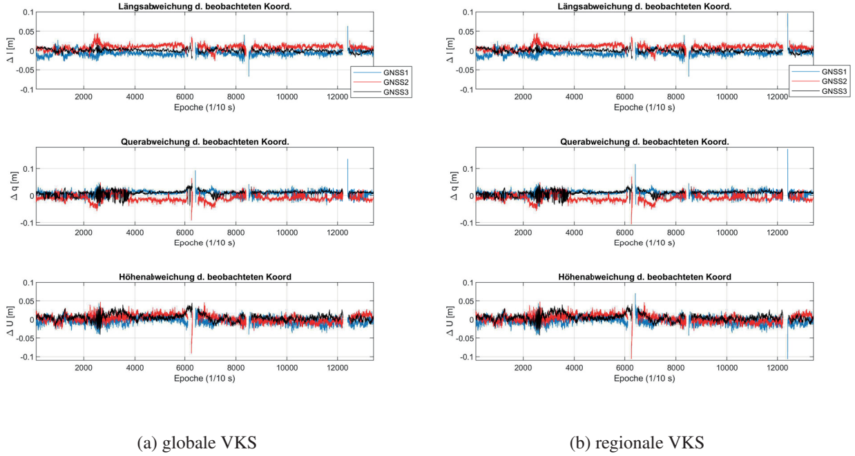
Abb. 5.9: Einfluss der geschätzten Varianzkomponenten auf die innovationen-basierten Längs- und Querabweichungen und d_{U,GNSS,k+1} bei der Modellerweiterung KINEMATIK (Szenario 3)
