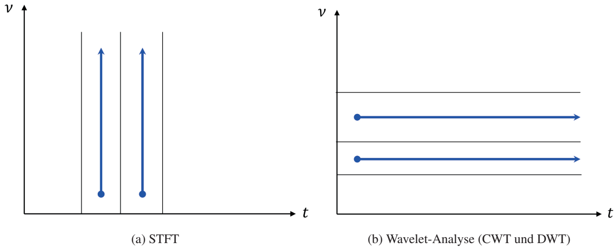
Abb. 3.13: Betrachtungsrichtung eines einzelnen Analyseschritts der Fourier-Transformation und der Wavelet-Analyse
