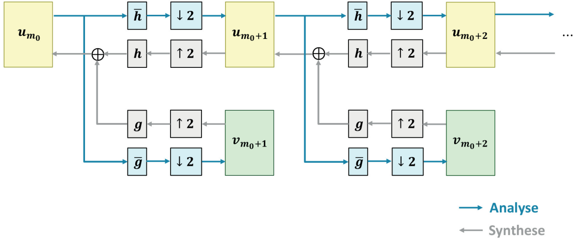
Abb. 3.10: Schnelle Wavelet-Transformation - Analyse und Synthese durch Filterung des Signals (nach Bani 2005; Mallat 2009)
