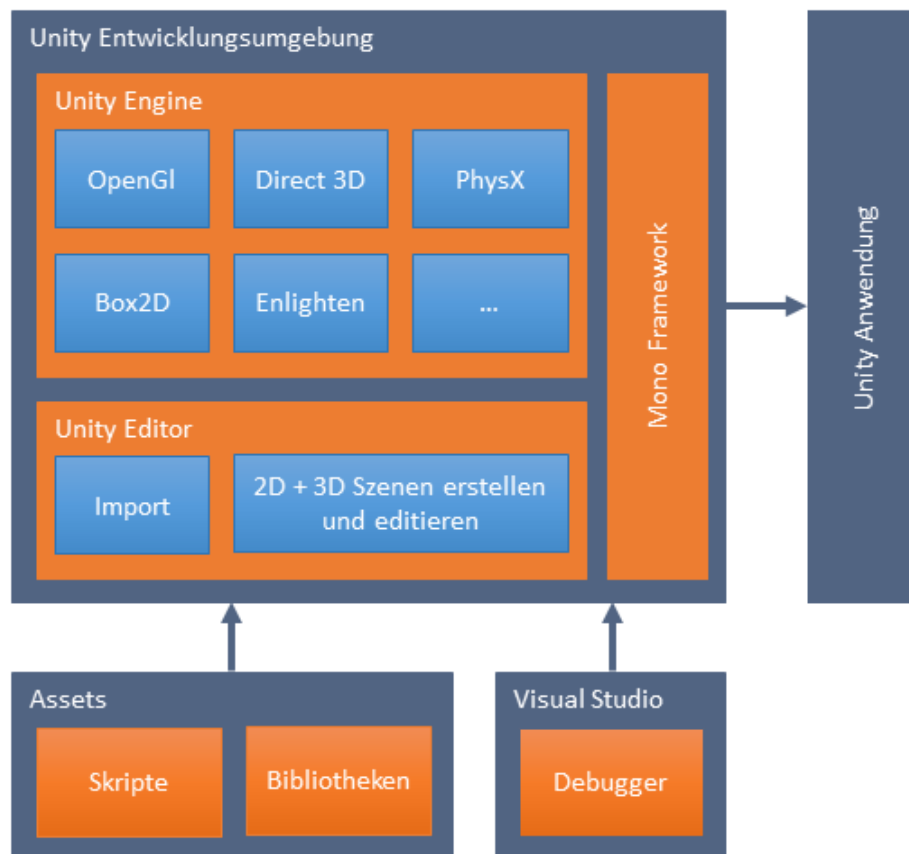
ABBILDUNG 8 - ABSTRAKTER AUFBAU DER KOMPONENTEN DER UNITY ENTWICKLUNGSUMGEBUNG
