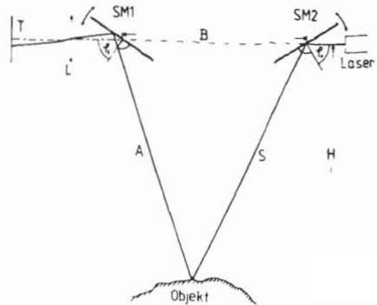
Bild 2: Erweiterter Aufbau zur zweiachsigen Oberflächenvermessung
