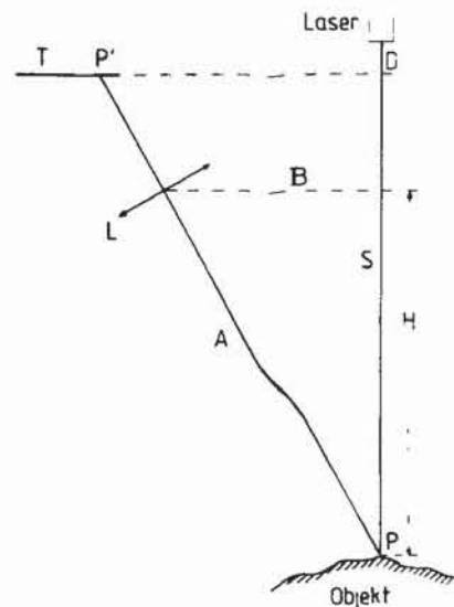
Bild 1: Standardaufbau zur Abstandsmessung durch optische Triangulation
