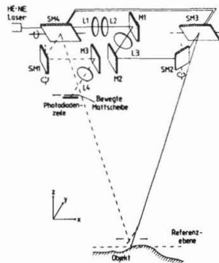
Bild 3: Realisierter Aufbau zur dreiachsigen Oberflächenvermessung
